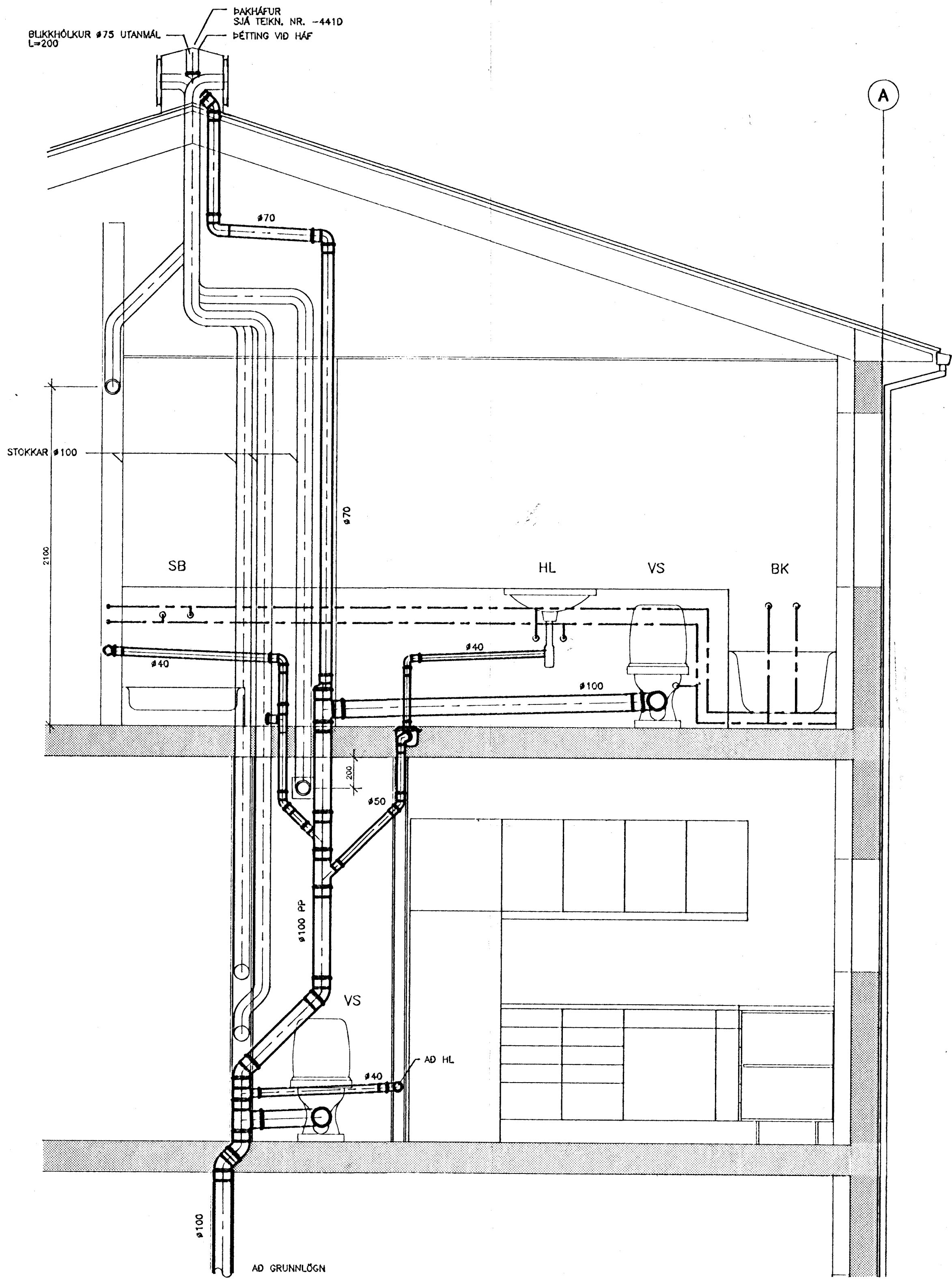
LAGNIR Í LAGNAVEGGJUM, 1:20
