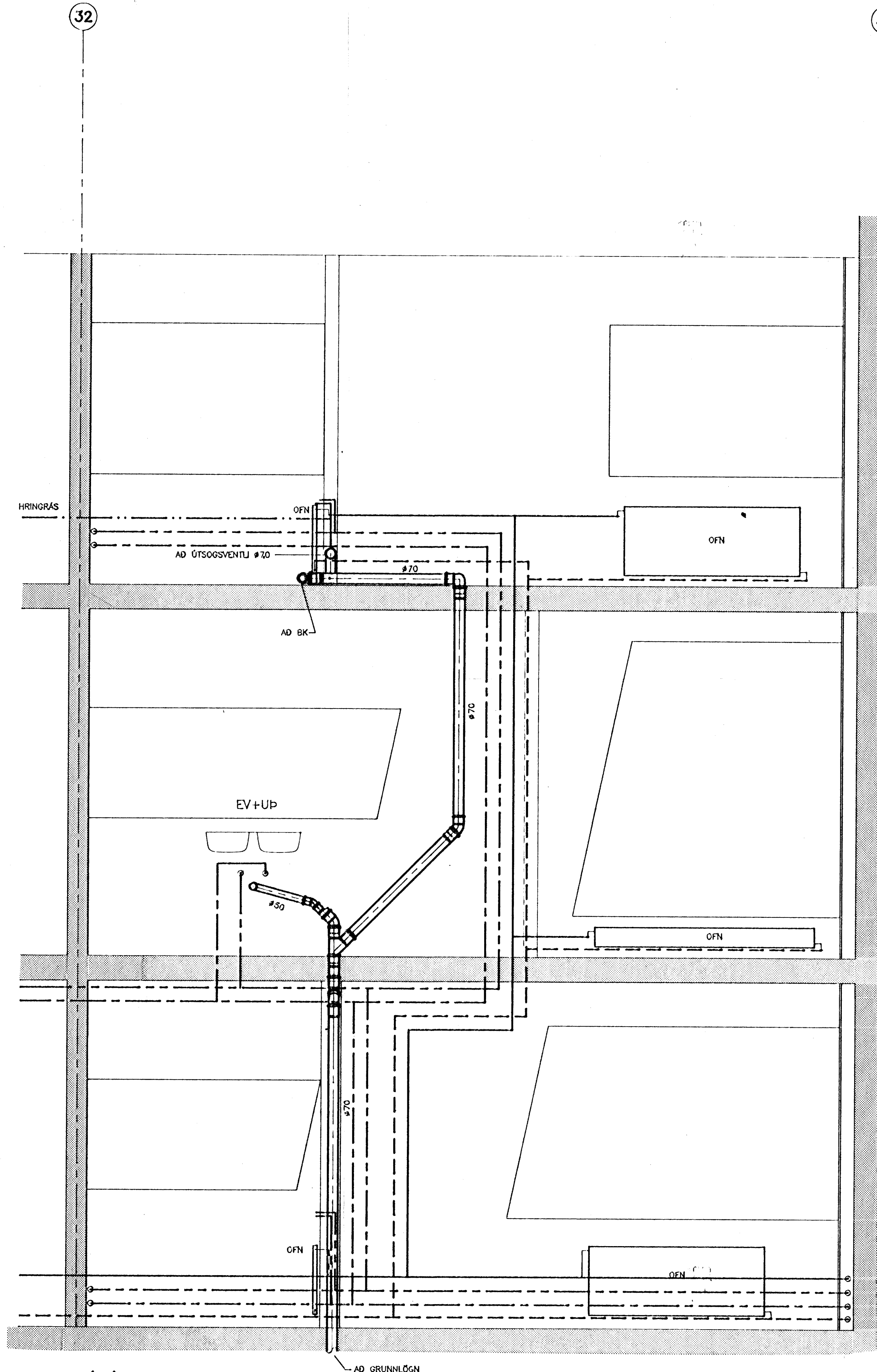
LAGNIR Í ÚTVEGG, 1:20
