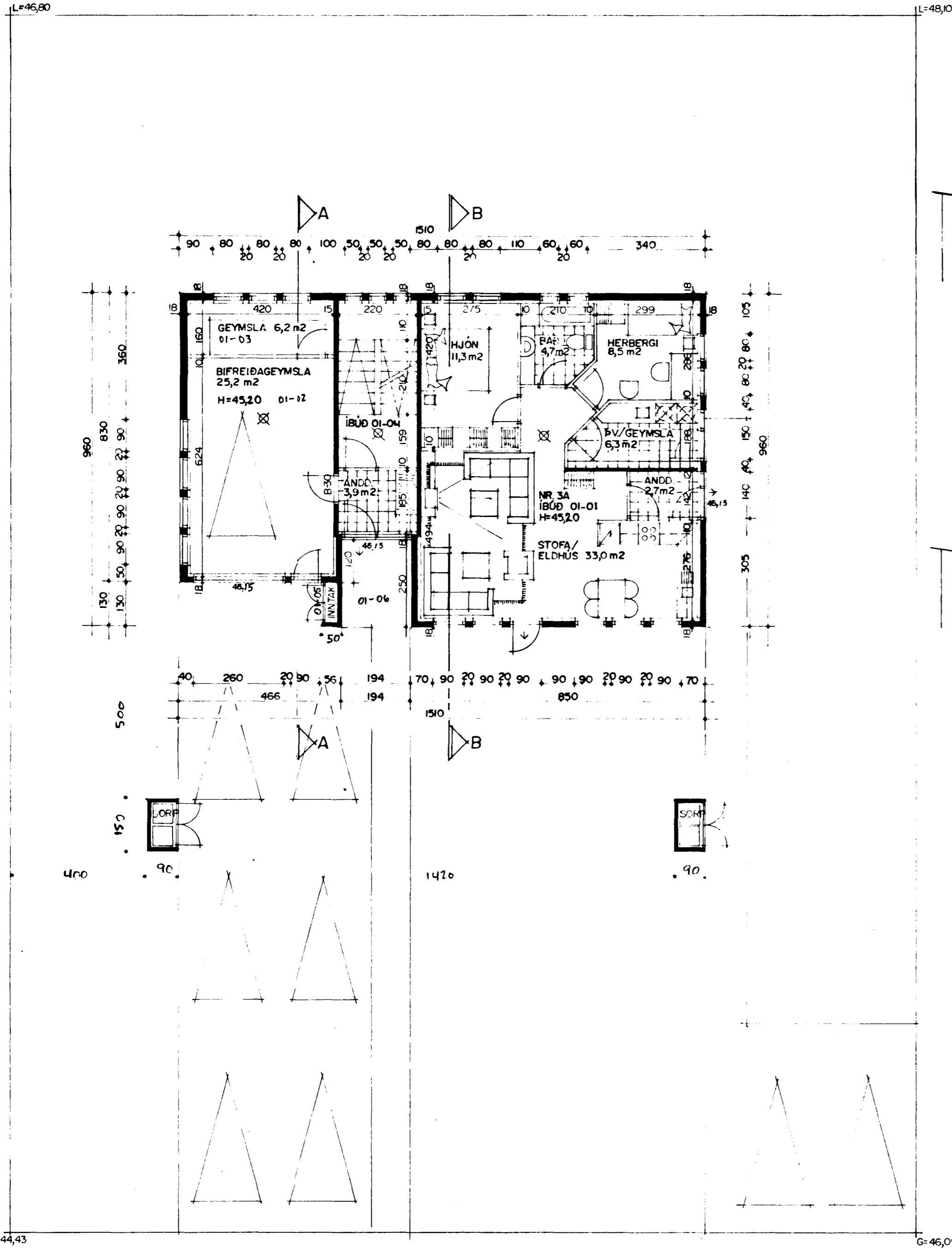
GRUNNMYND I HÆÐ MKV. 1:100
