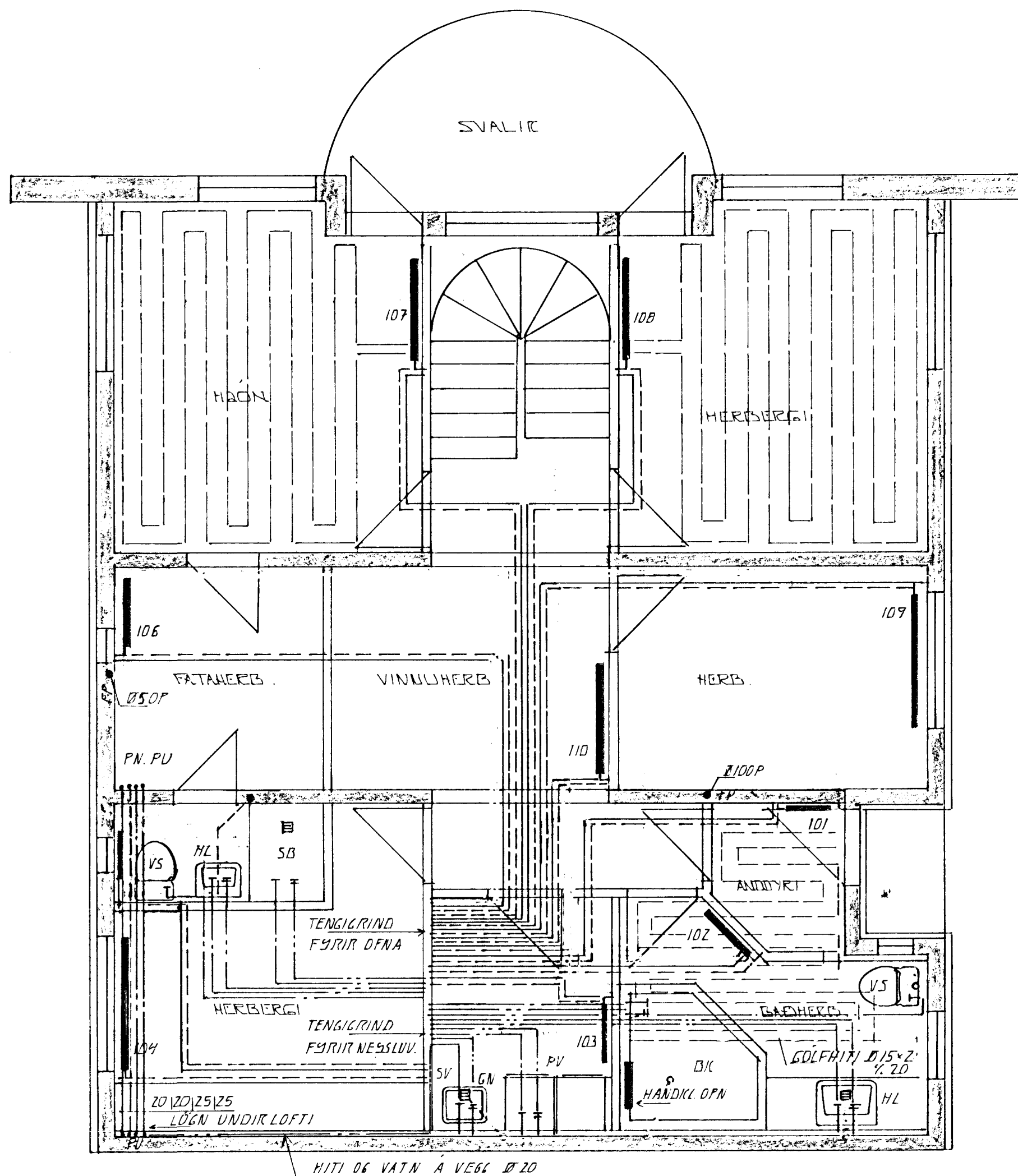
GRUNNMYND NEDRI HEDAR 1:50
