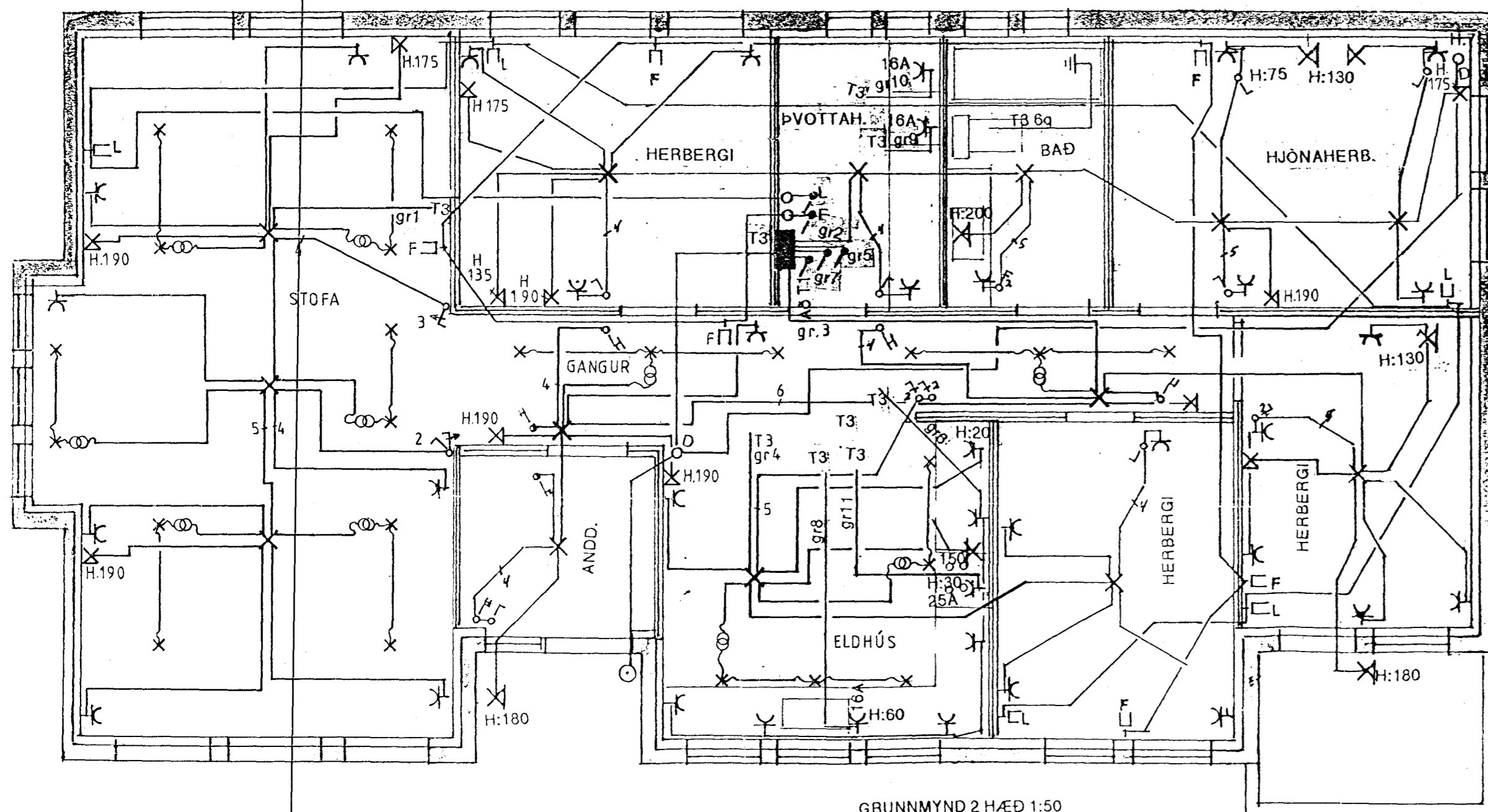
GRUNNMYND 2 HÆÐ 1:50
