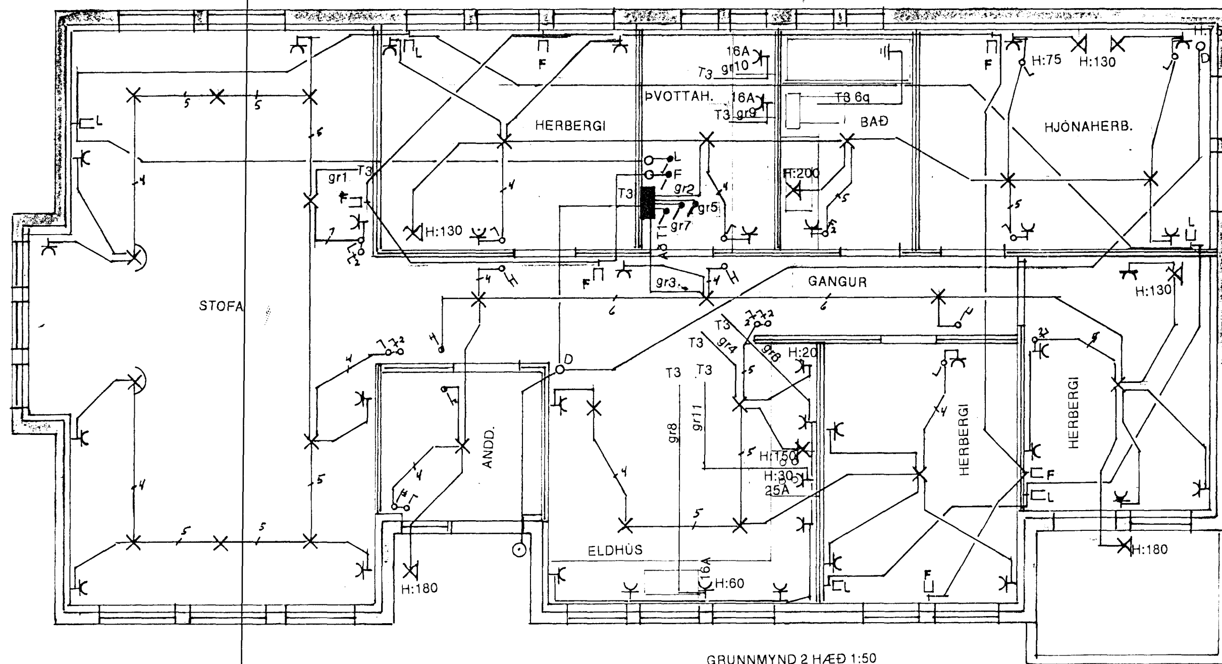
GRUNNMYND 2 HÆÐ 1:50
