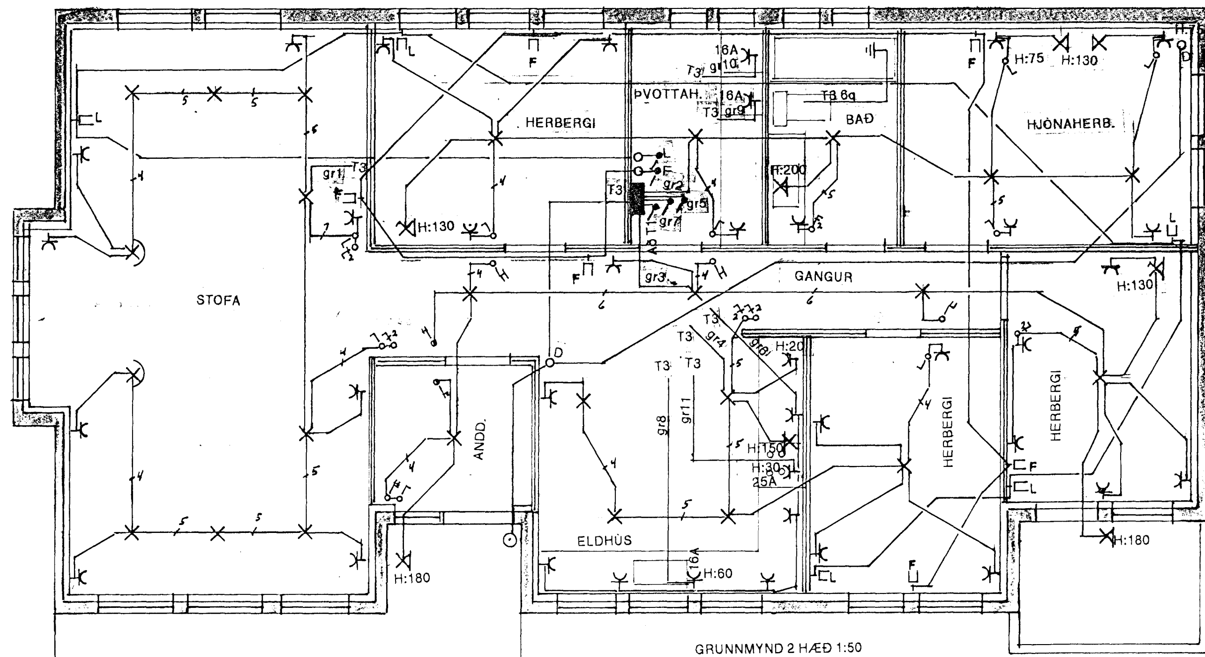
GRUNNMYND 2 HÆÐ 1:50
