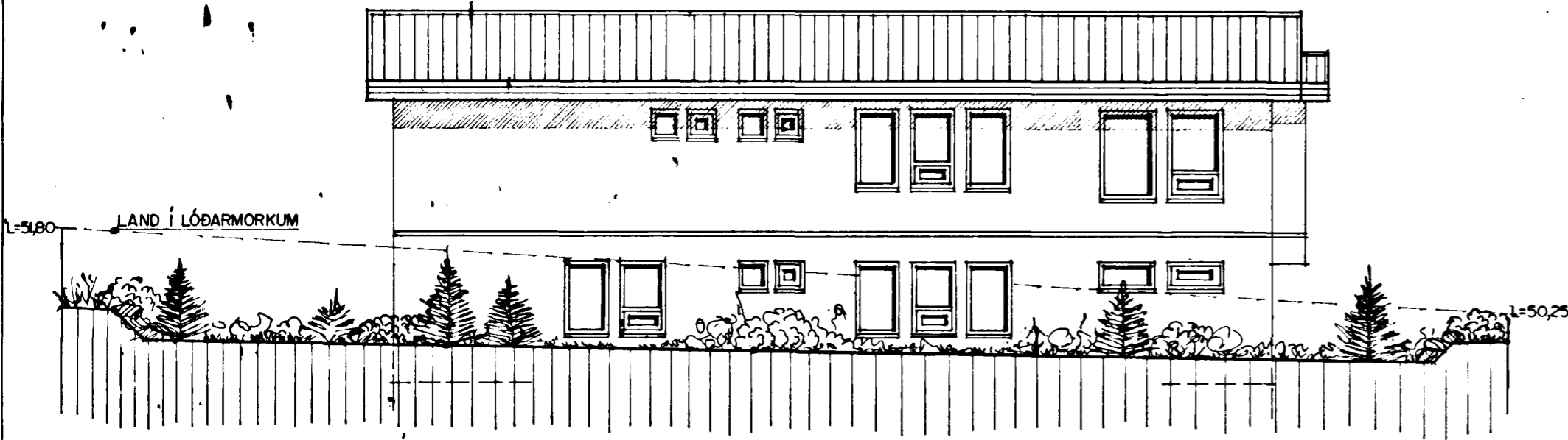
ÚTLIT NORÐAUSTUR MKV. 1:100.
