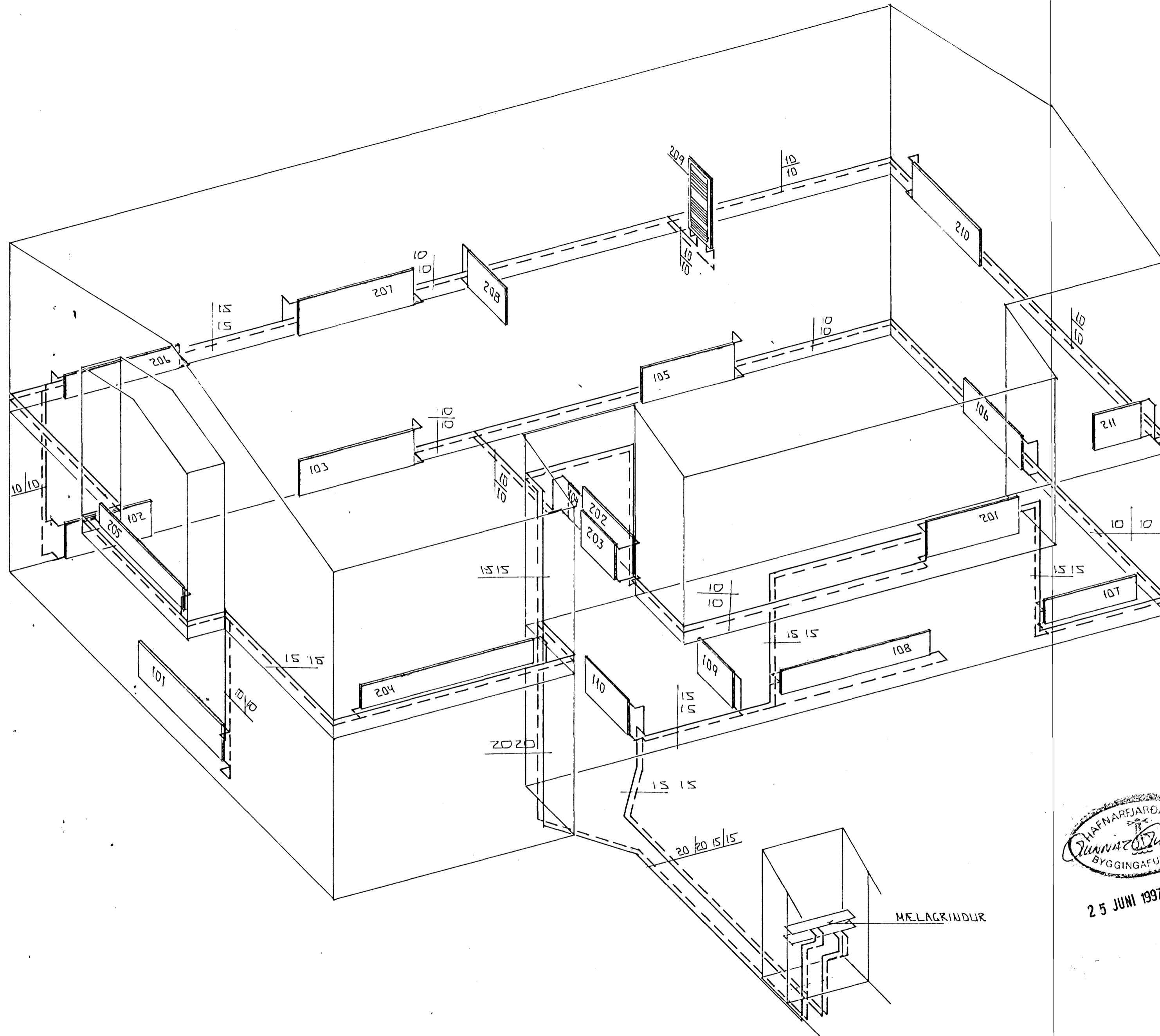
RÚMMYND - HITALAGNA 1:50
