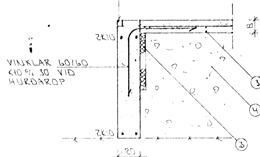
SNID 3 : 1 : 20
