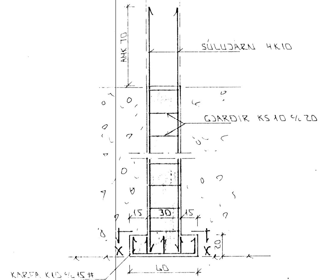
SNILA S1 : 1 : 20
