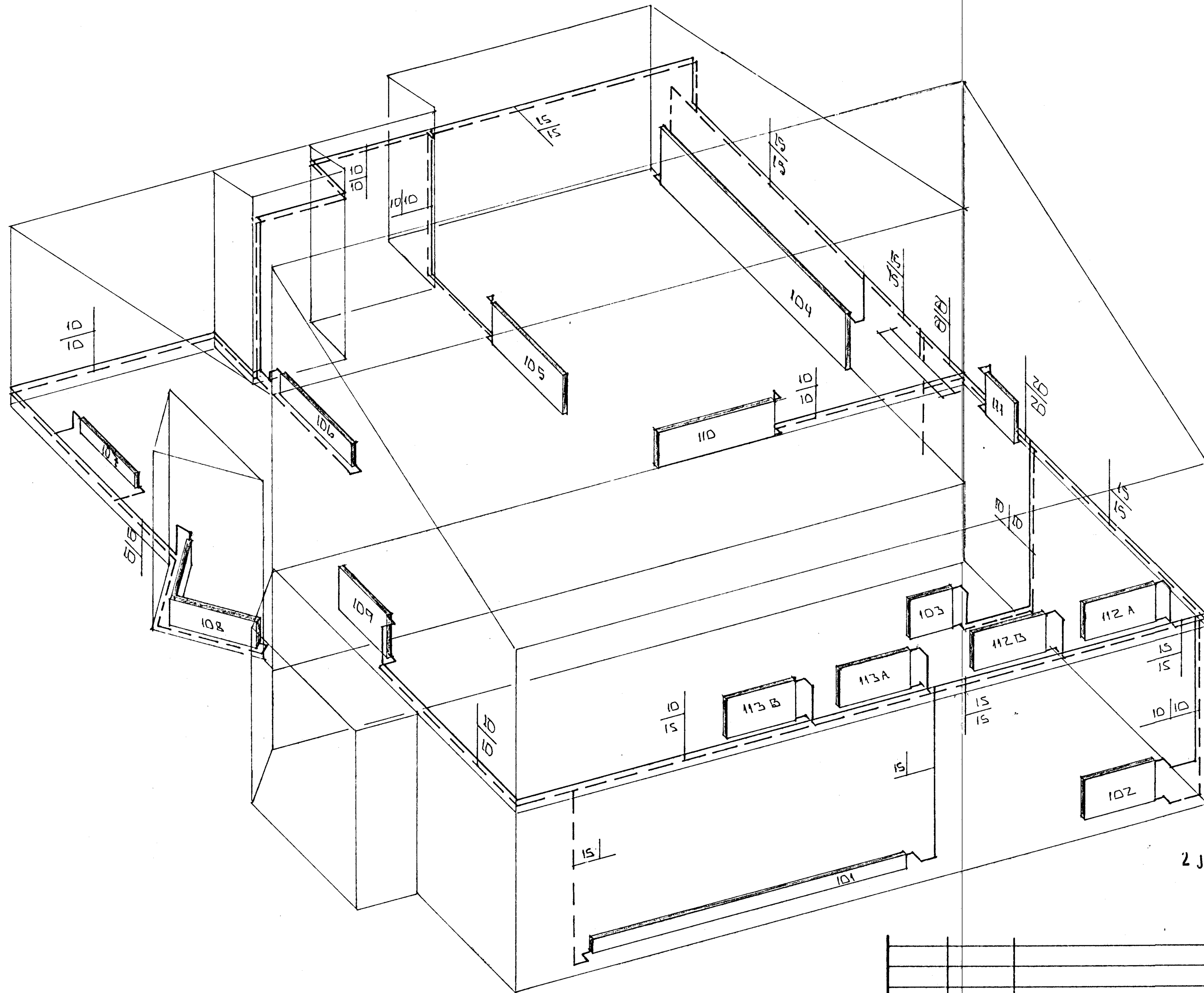
RÚMMYND HITALAGNA ~ 1:50
