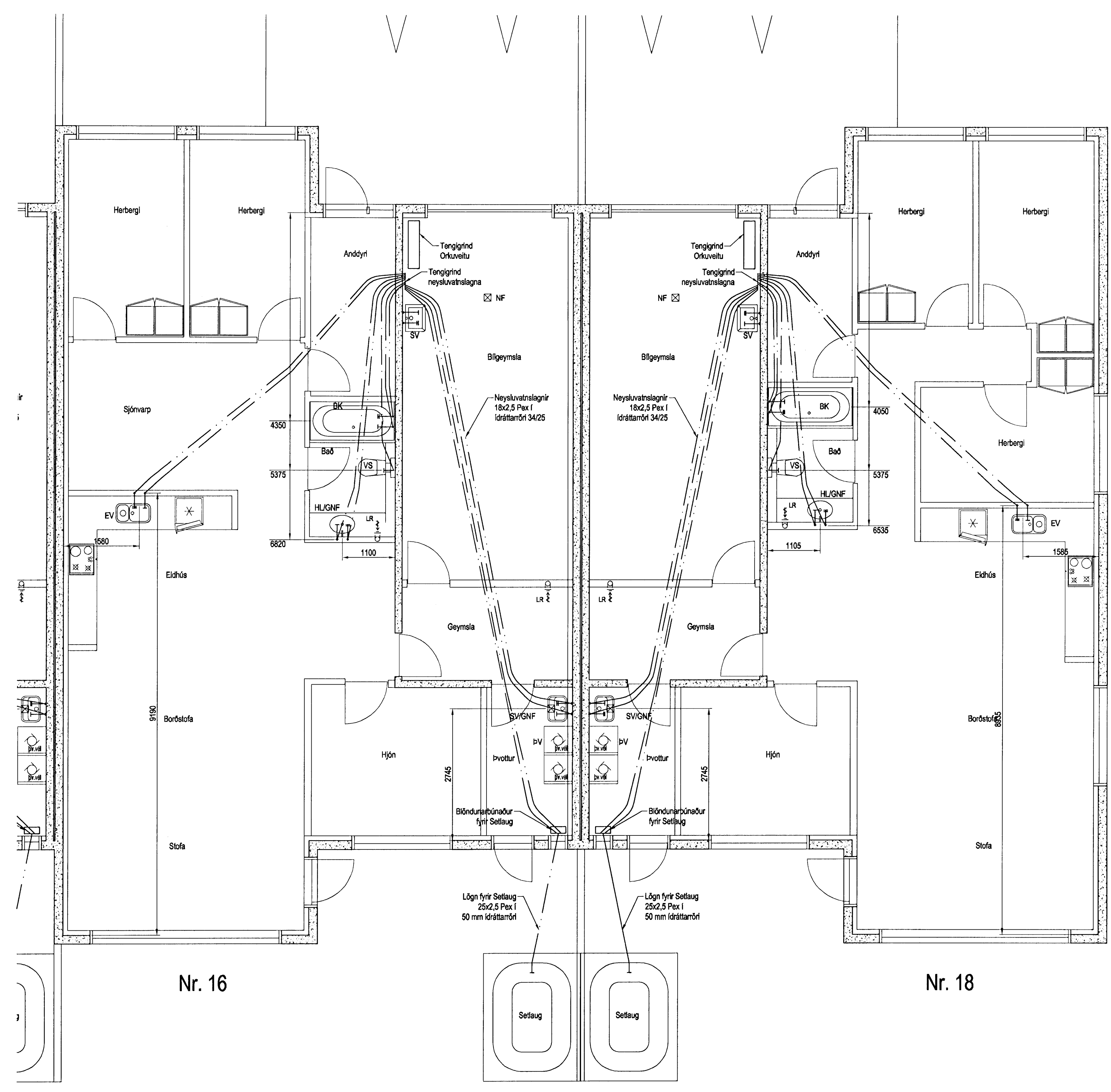
Neysluvatnslagnir, 1:50
