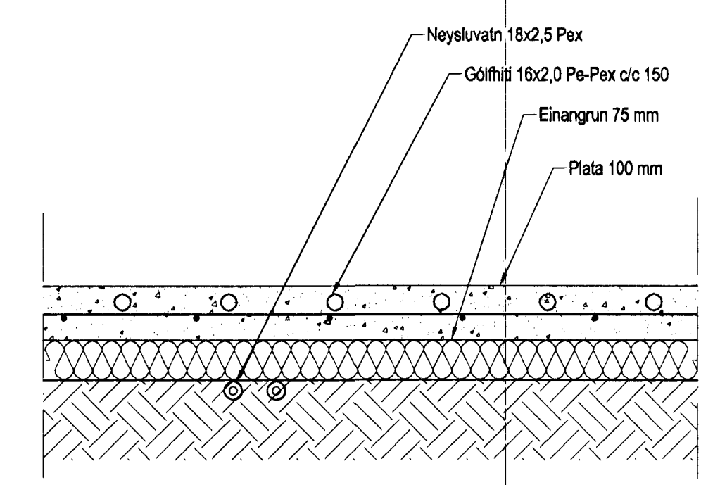
Hita- og vatnslagnir, Snið í botnplötu, íbúð 1:10
