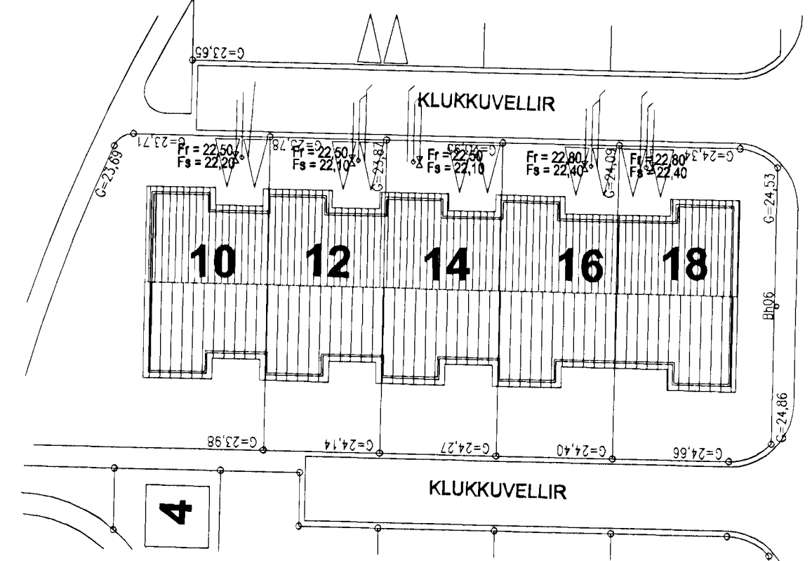
Afstöðumynd, 1:500
