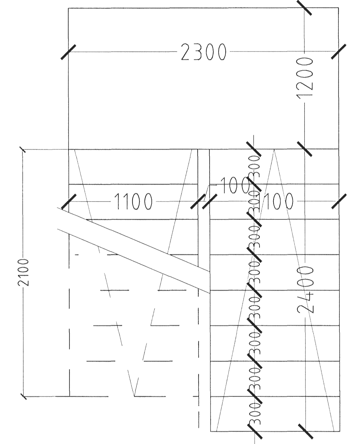
HLUTAMYND STIGI MKV. 1:20.
