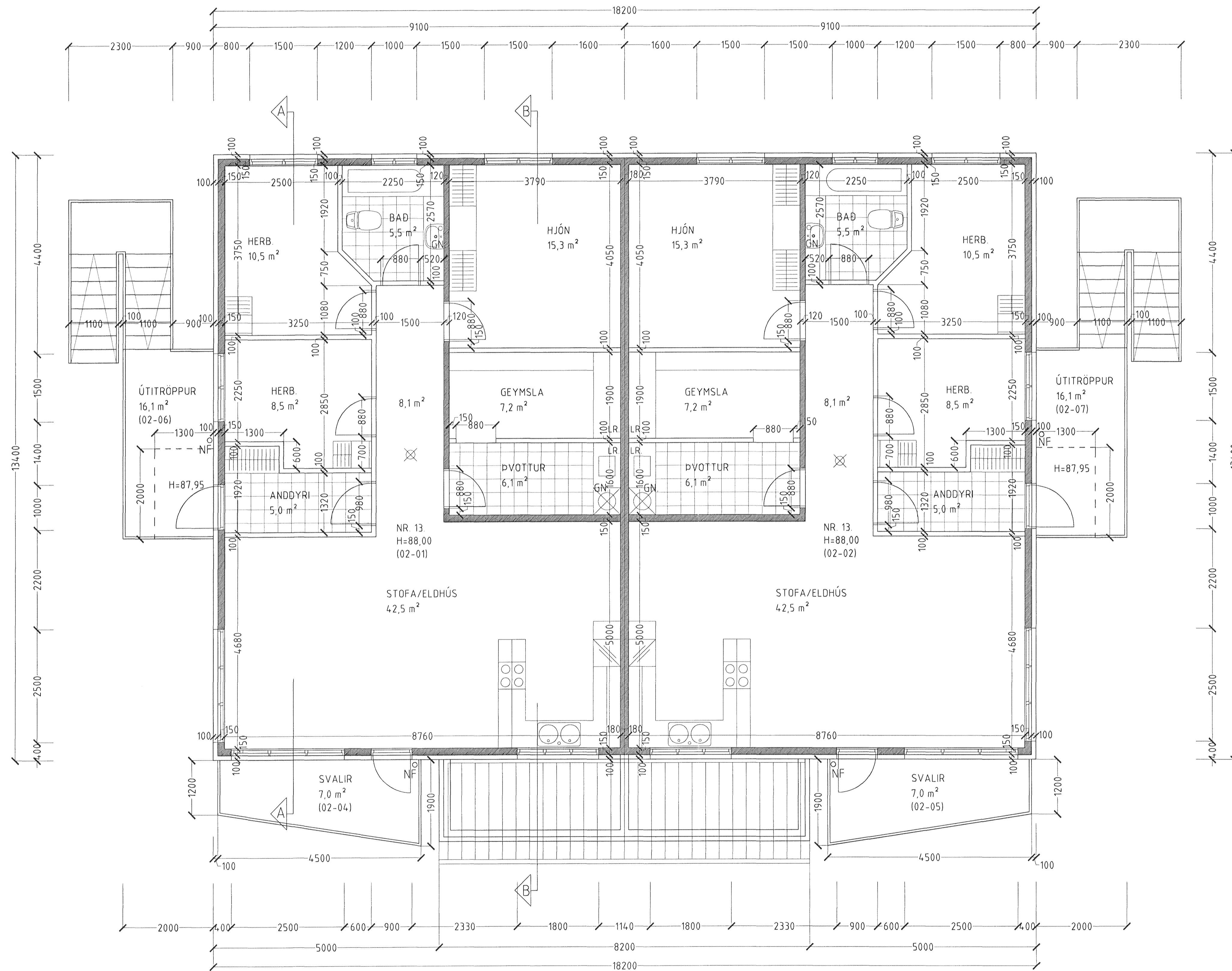
GRUNNMYND 2 HÆÐ MKV. 1:50.
