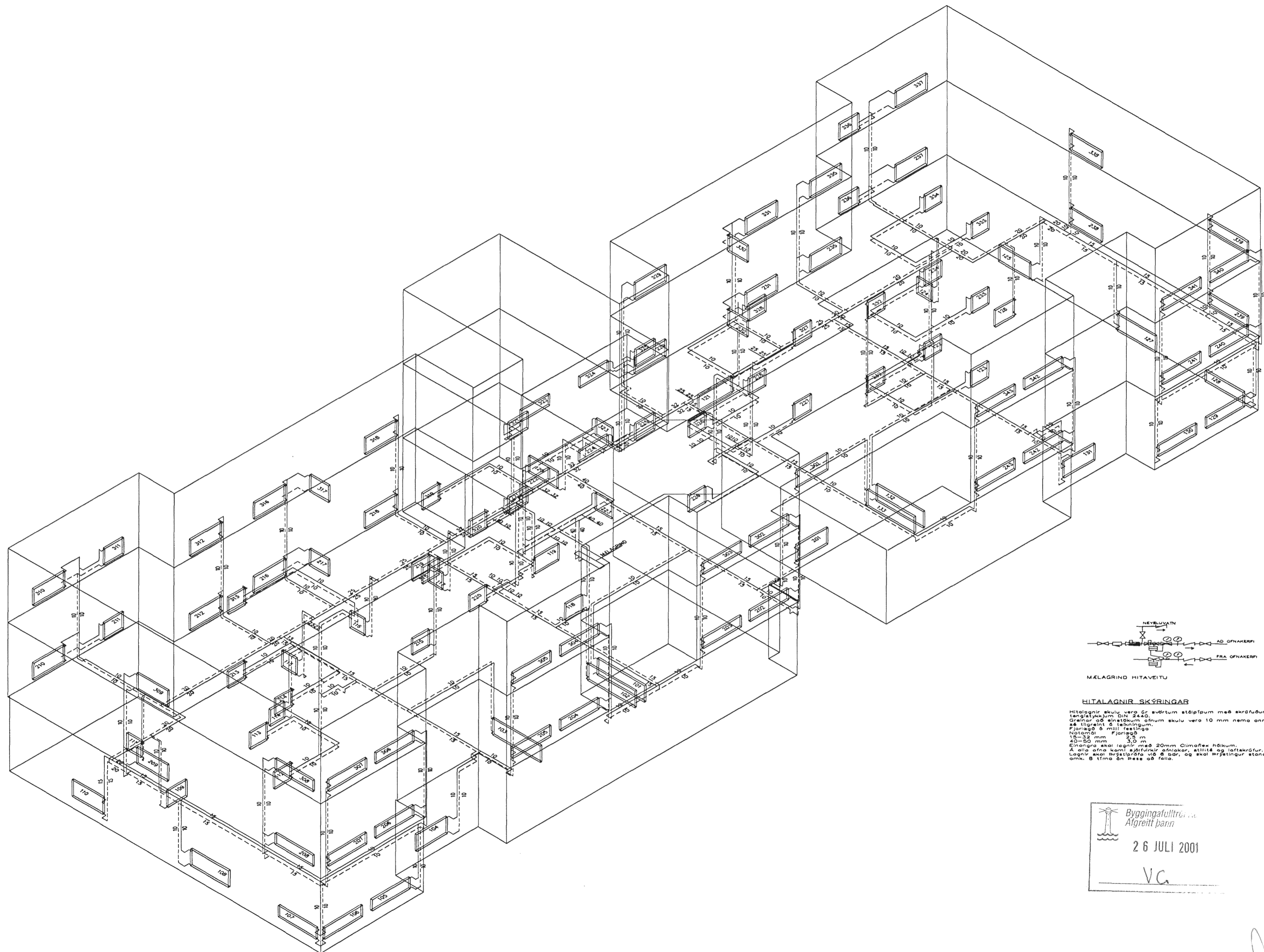
RÚMMYND HITALAGNA 1:100
