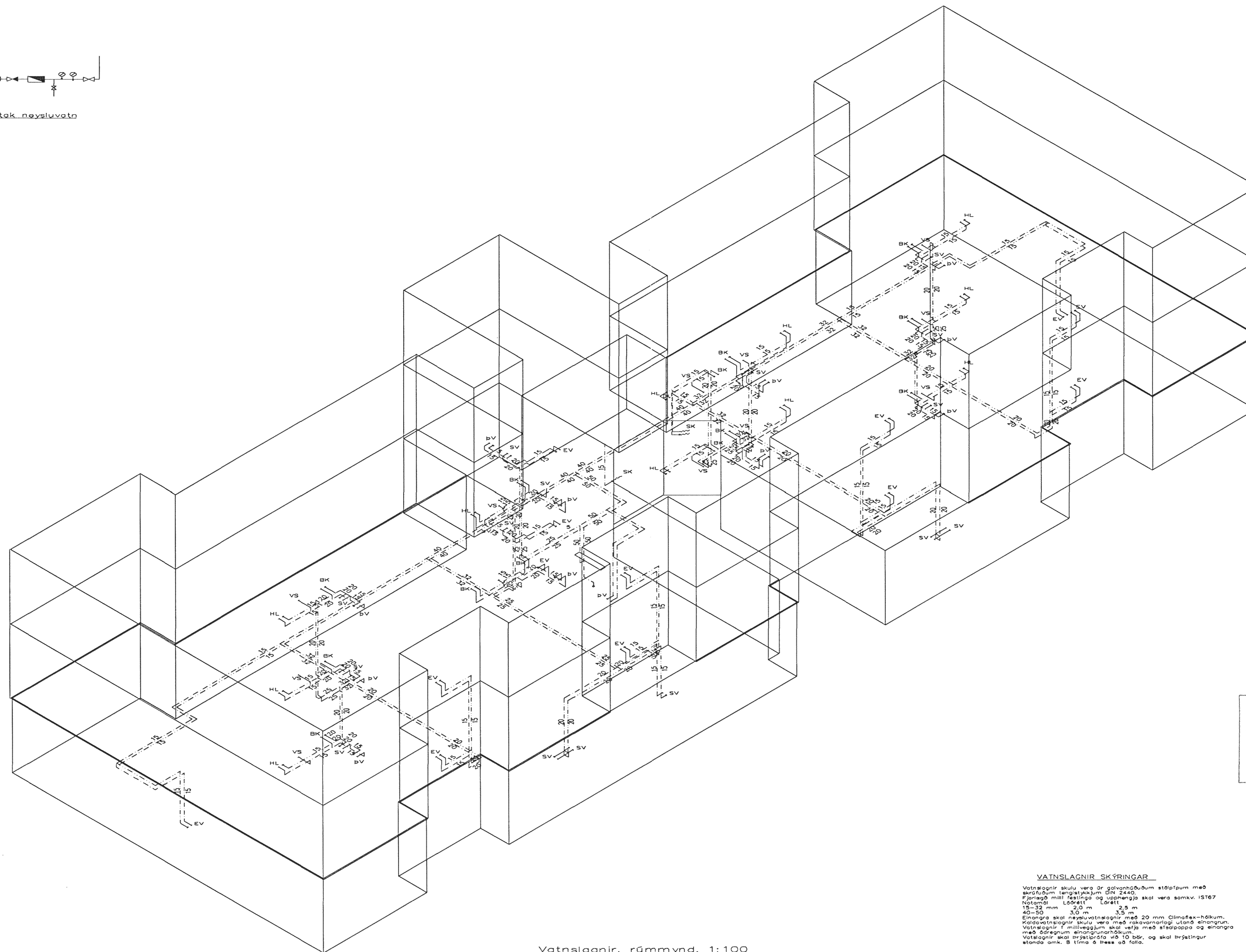
Vatnslagnir, rúmmynd, 1:100
