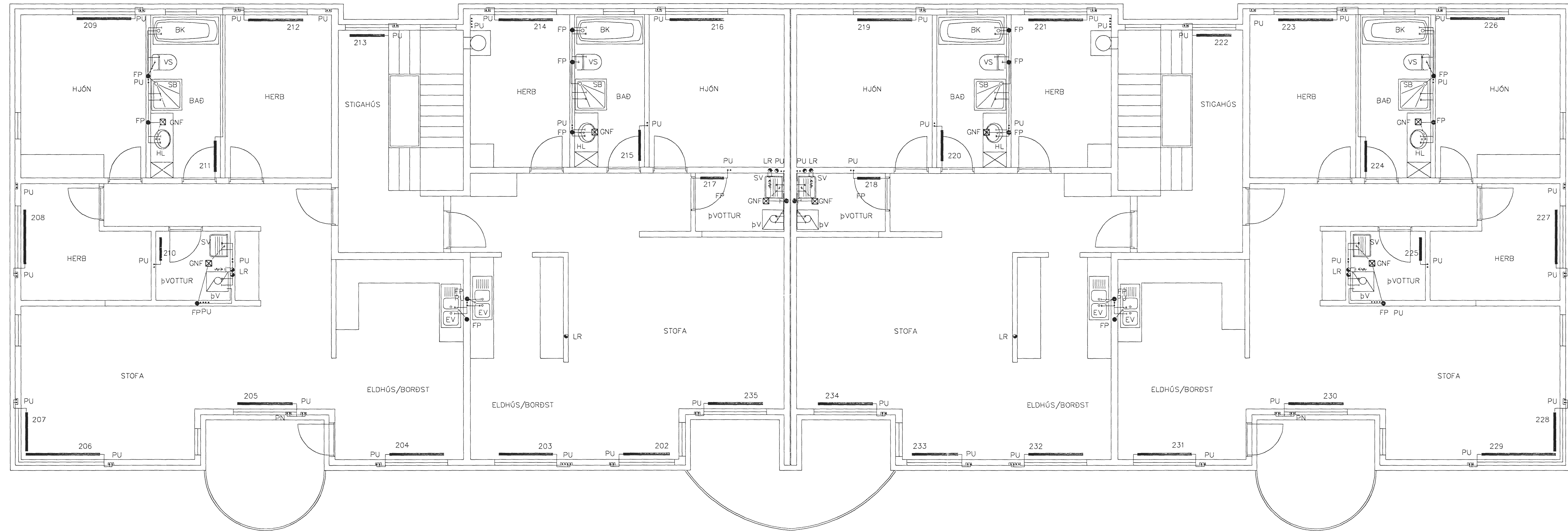
GRUNNMYND 2 HÆÐAR 1:50
