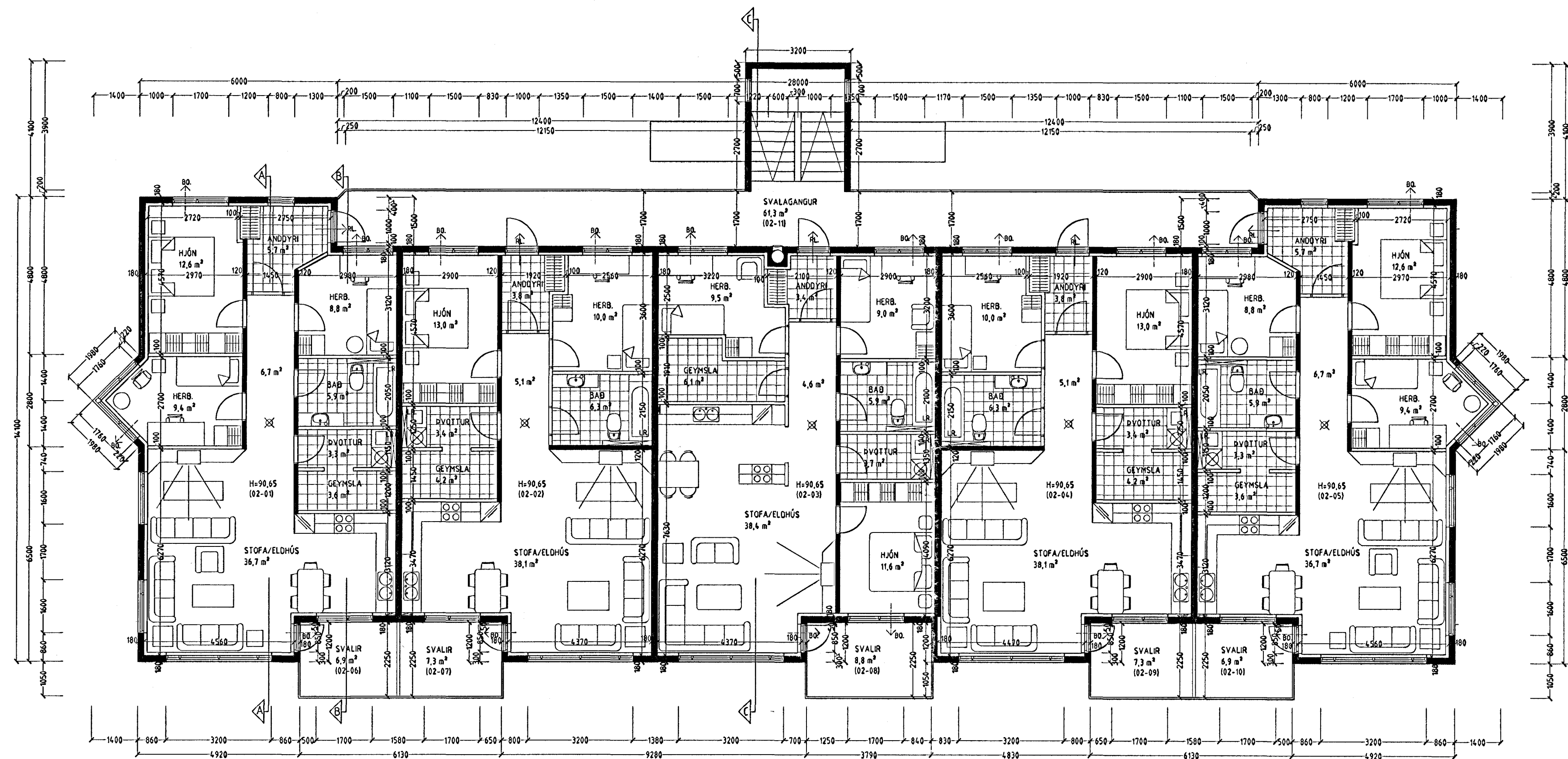
GRUNNMYND 2 HÆÐ MKV. 1:100.
