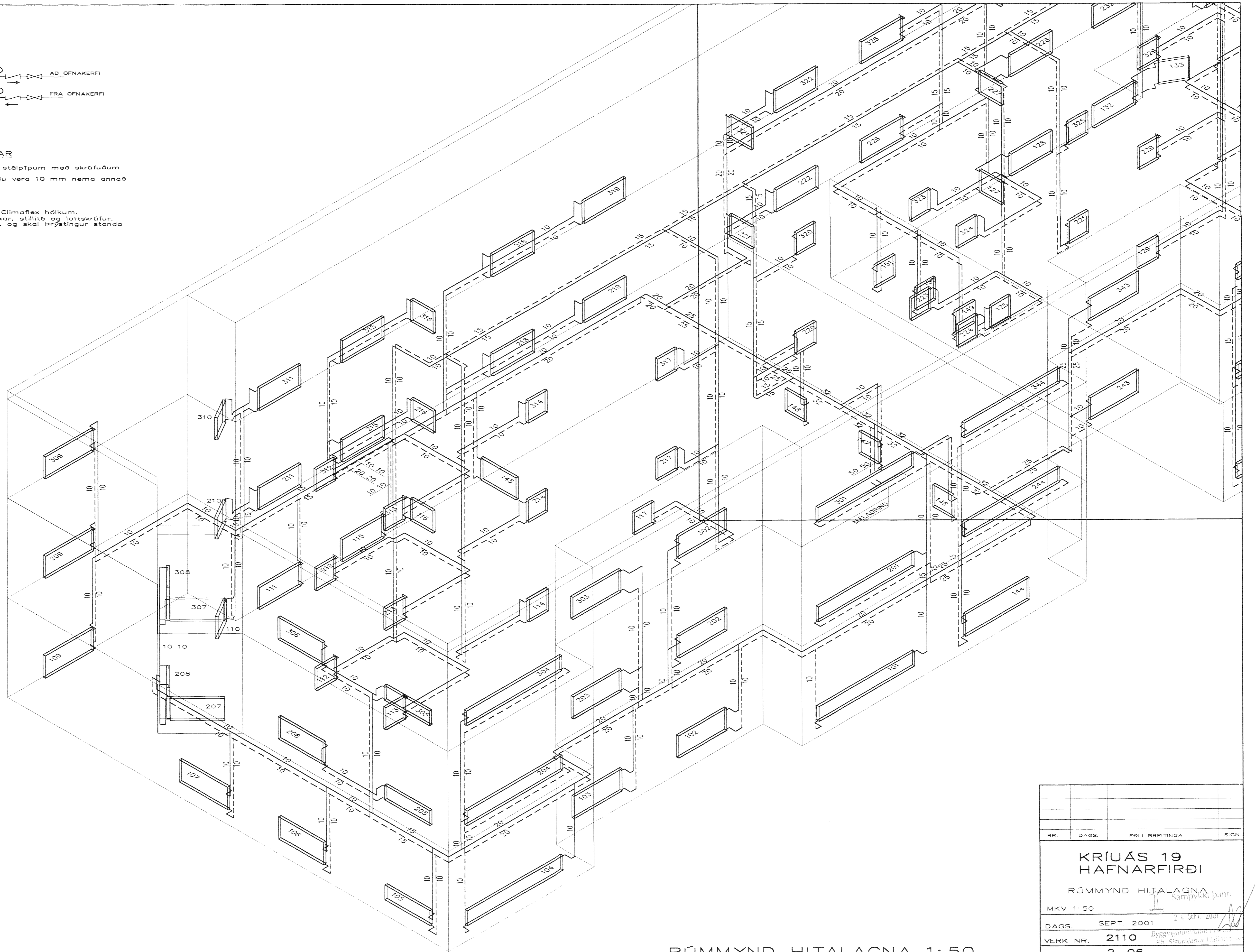
RÚMMYND HITALAGNA 1:50
