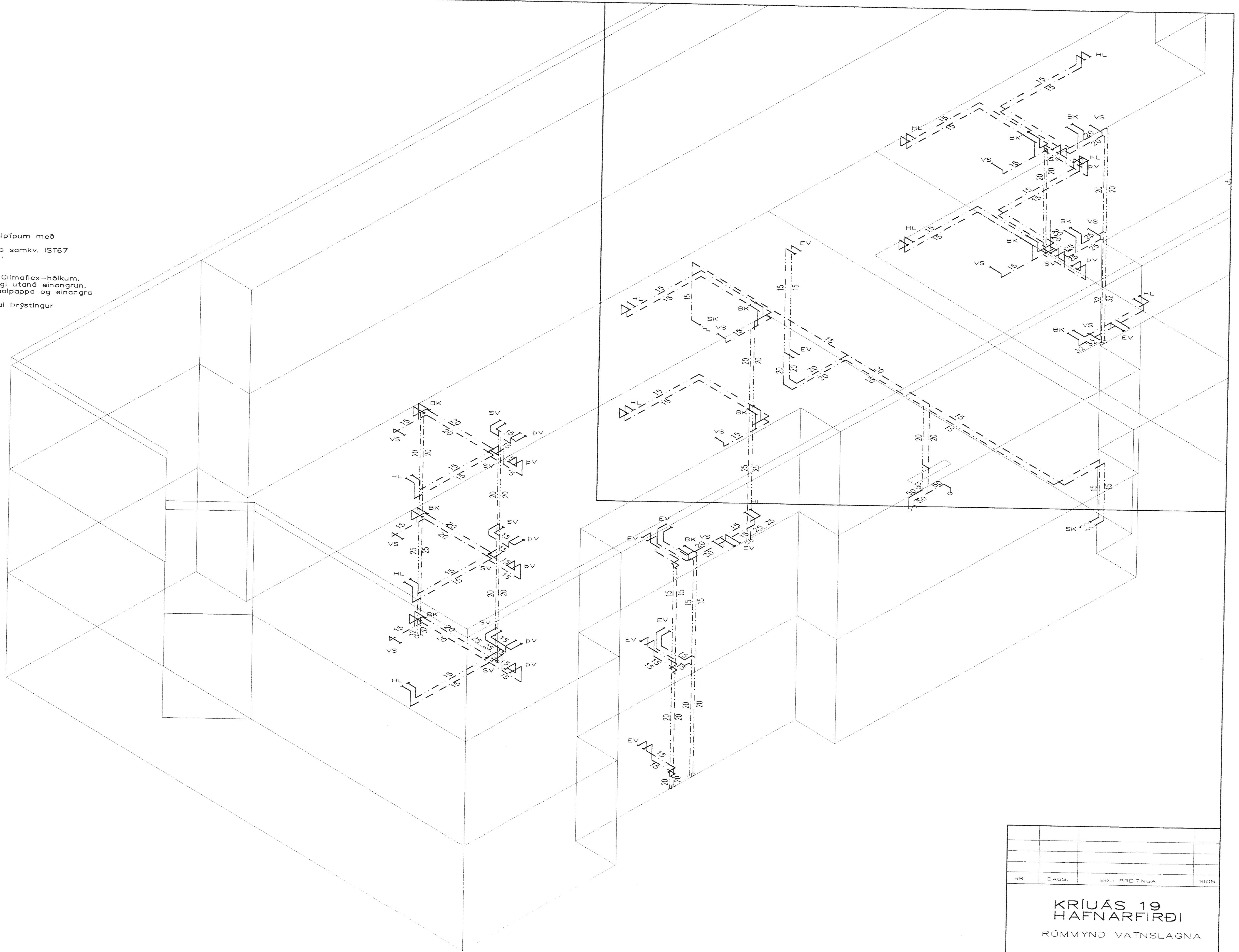
Vatnslagnir, rúmmynd, 1:50
