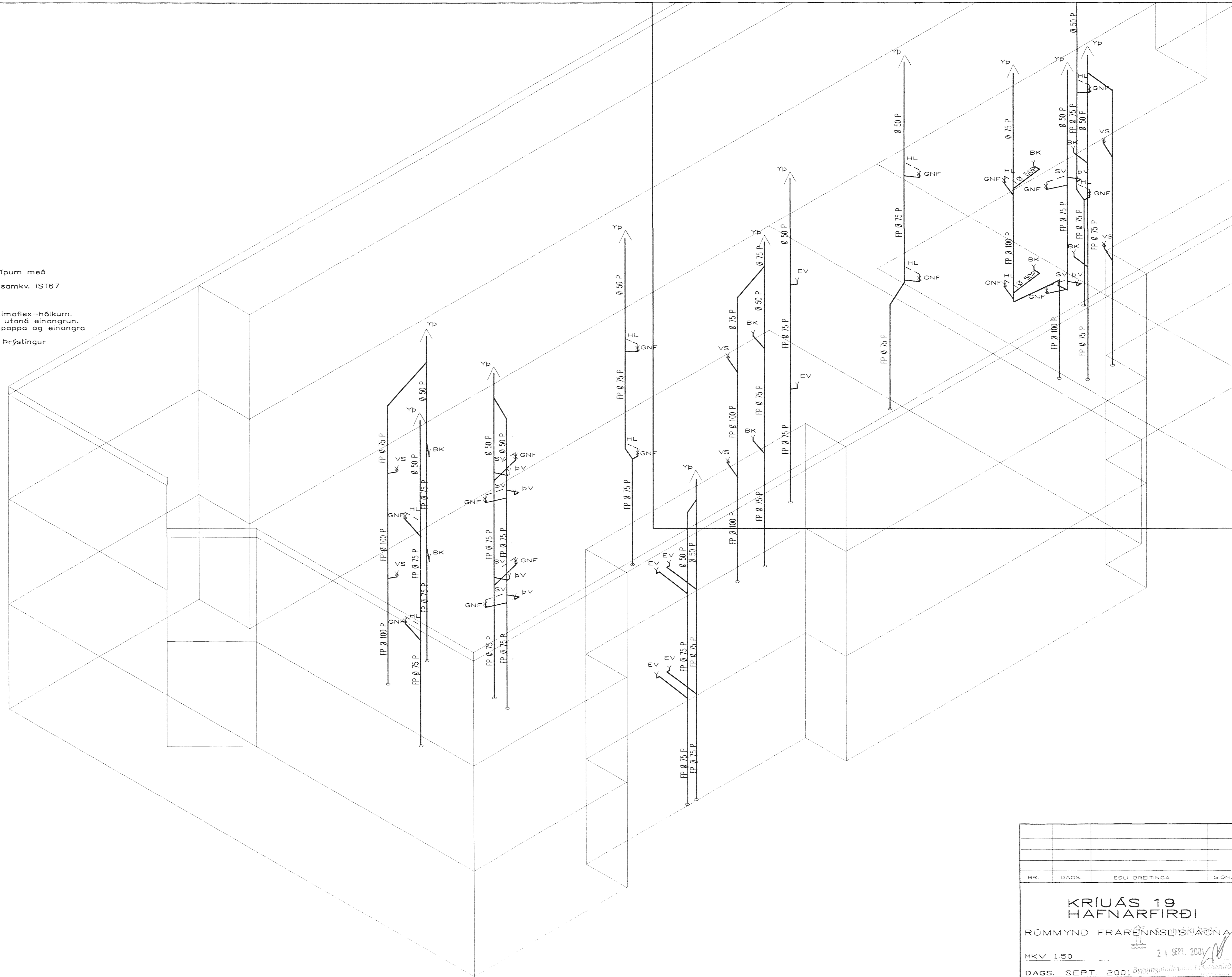
RÚMMYND FRÁRENNSLISLAGNA 1:50
