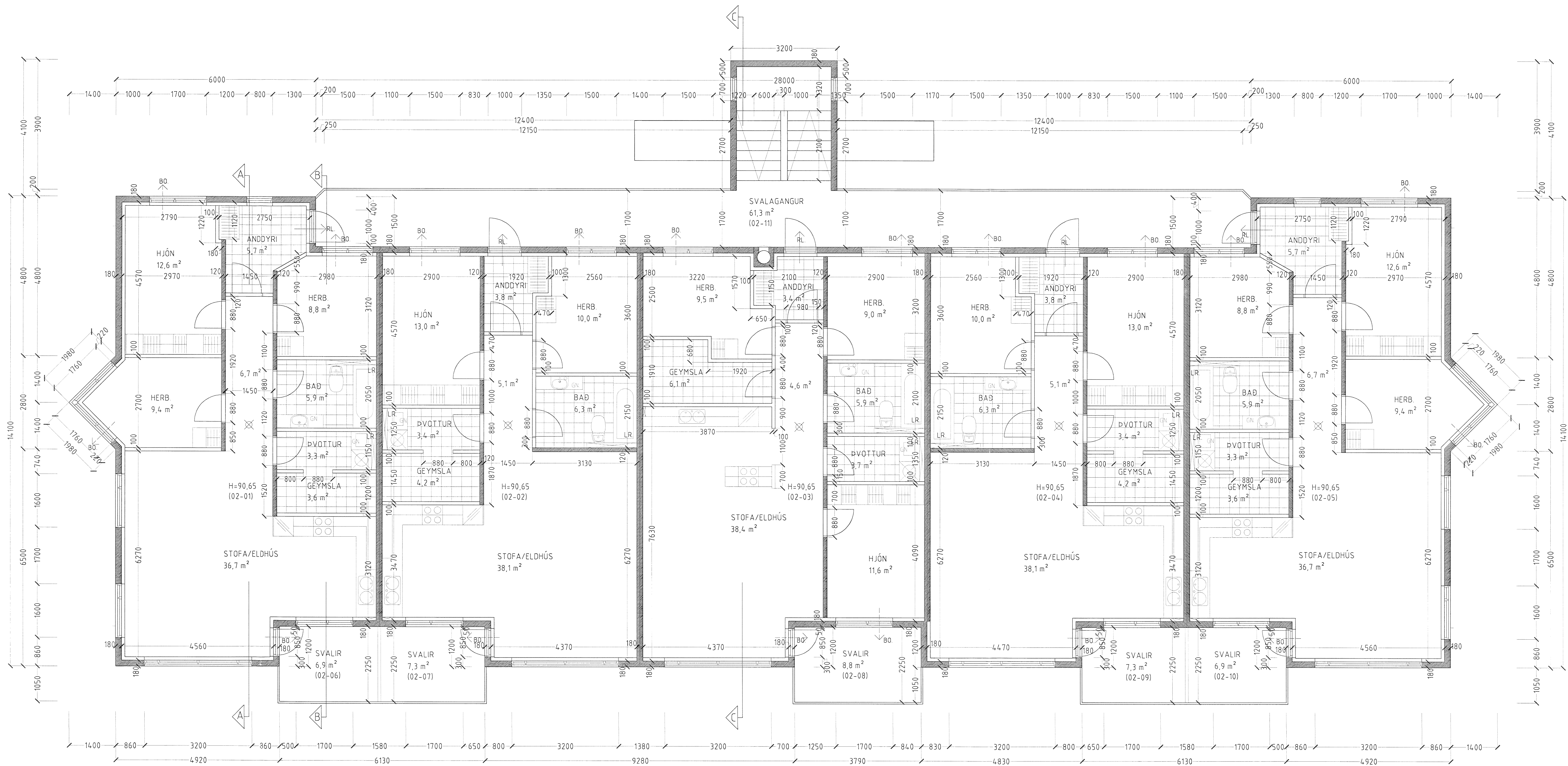
GRUNNMYND 2 HÆÐ MKV. 1:50.
