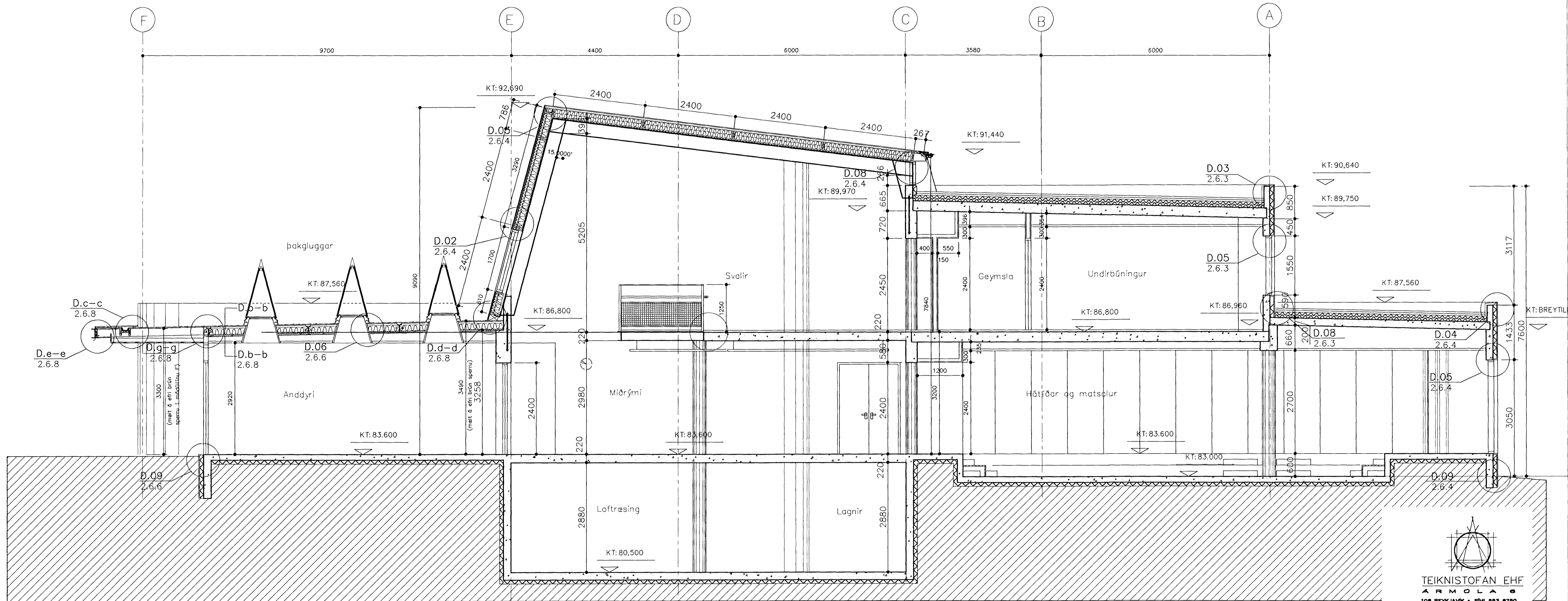
SNEIÐING B-B MKV, 1:50
