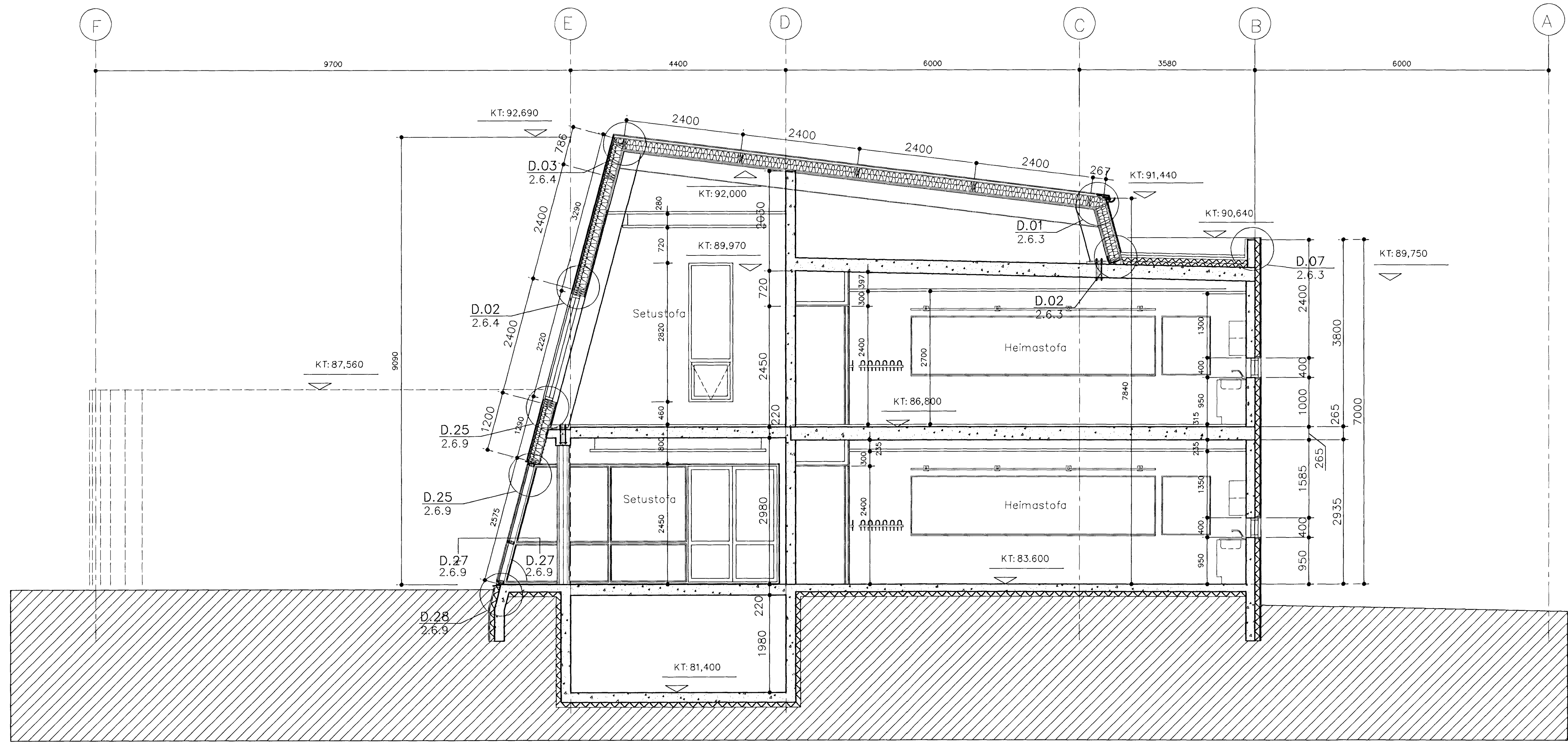
SNEIÐING G-G MKV, 1:50
