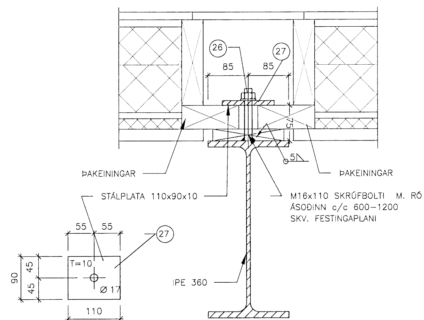
FESTINGAR FYRIR ÞAK- OG VEGGEININGAR 1:5
