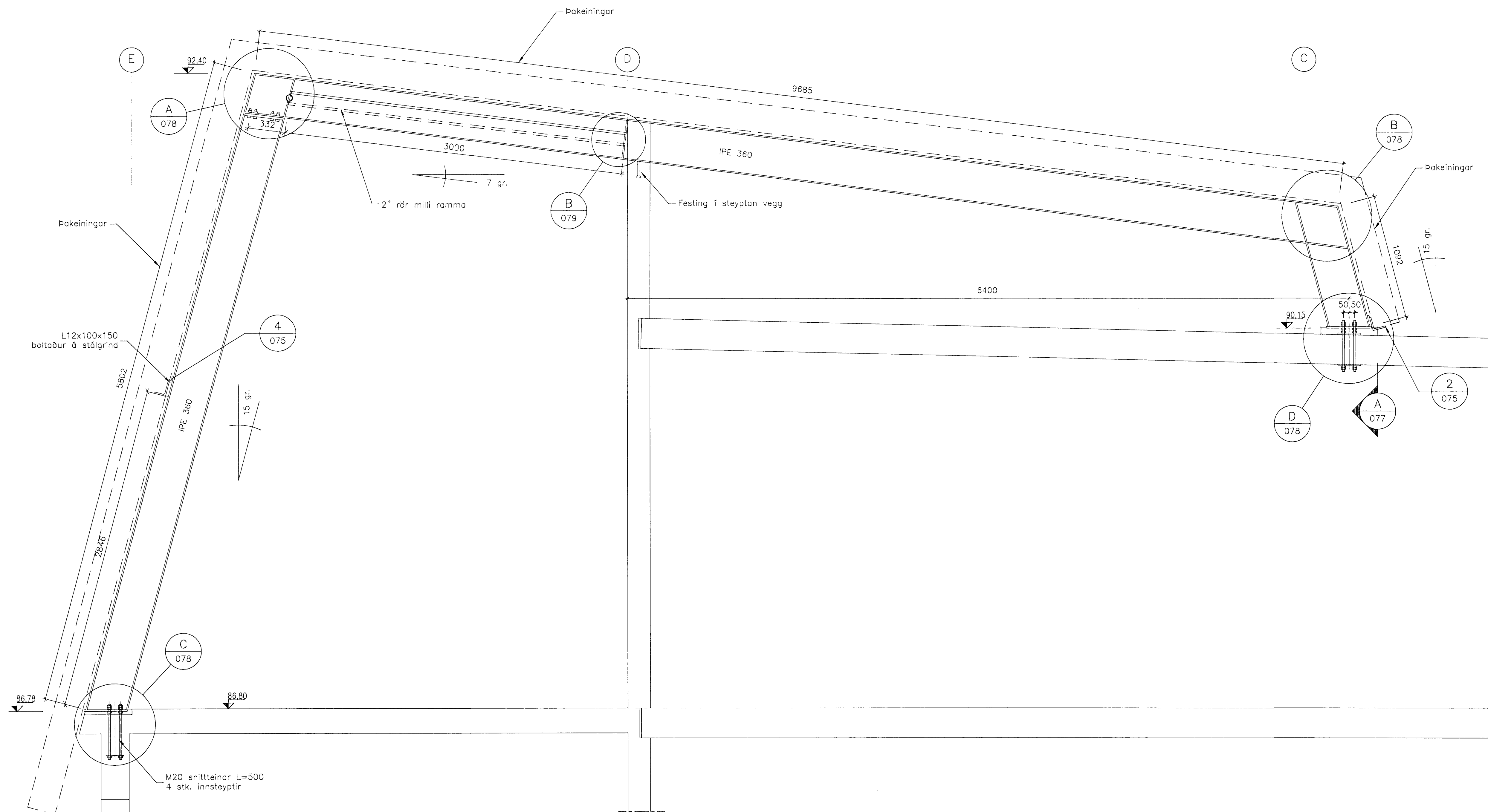
C SNID - STÁLRAMMAR NR. 3 1:20
