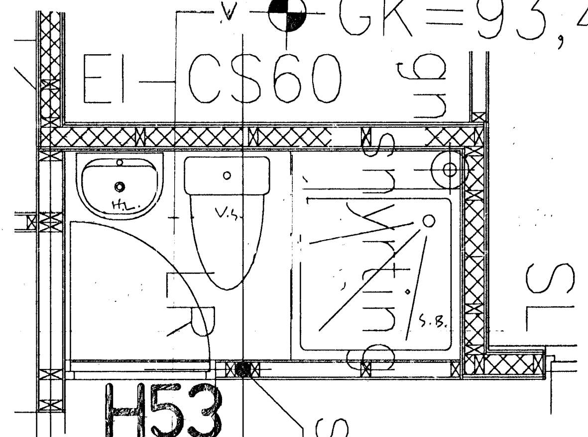
Snyrting grunnmynd mkv. 1:20
