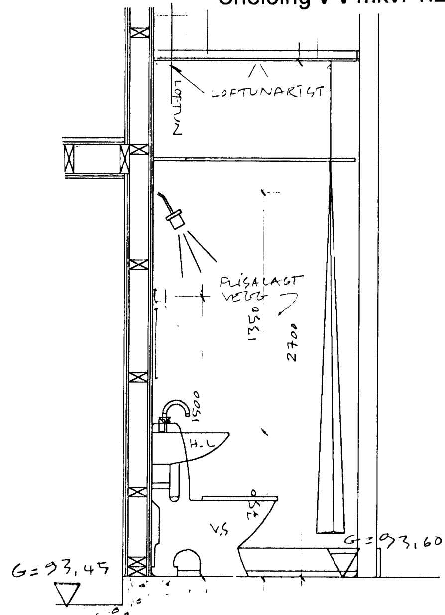
Sneiðing v-v mkv. 1:20
