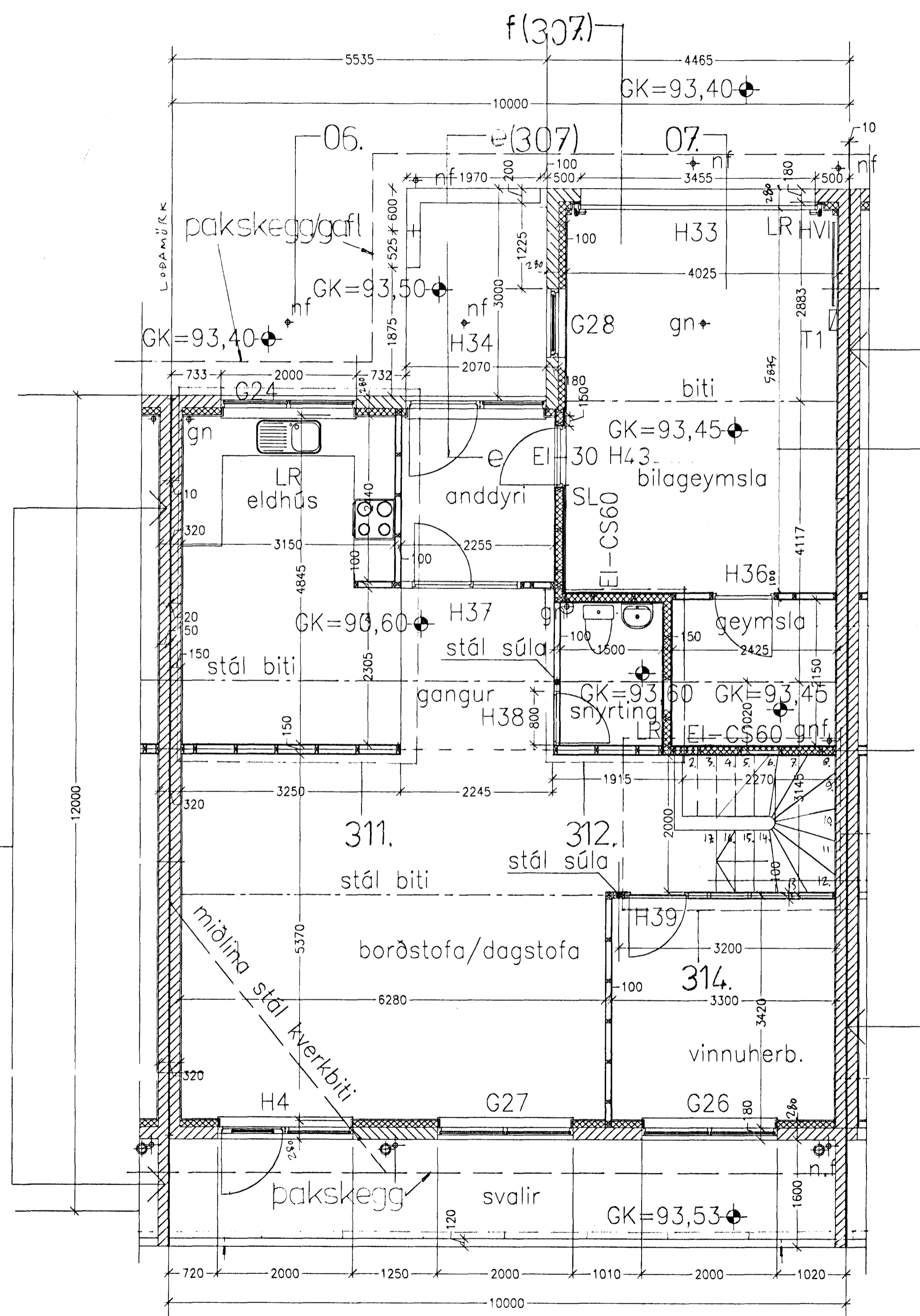
Grunnmynd 1.hæð mkv.1:50
