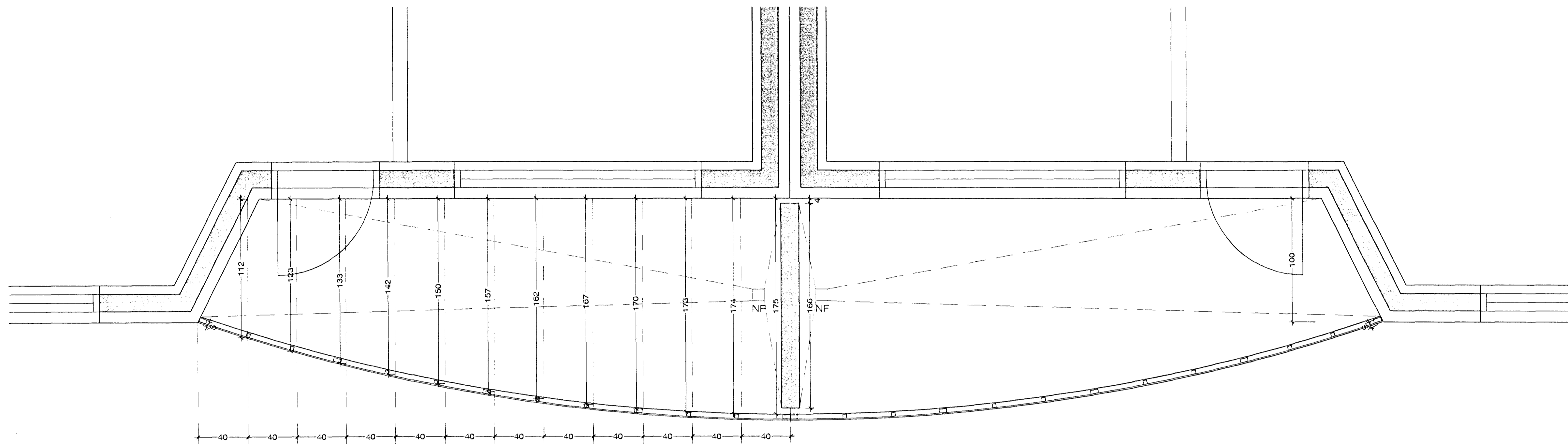
GRUNNMYND SVALIR M 1 : 20 Kriúás 39-41
