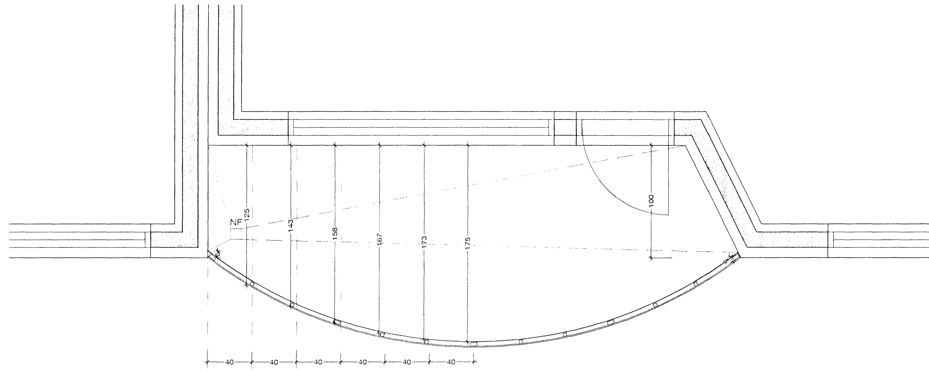
GRUNNMYND SVALIR M 1 : 20 Kríuás 37 (Kríuás 43 spegilmynd)
