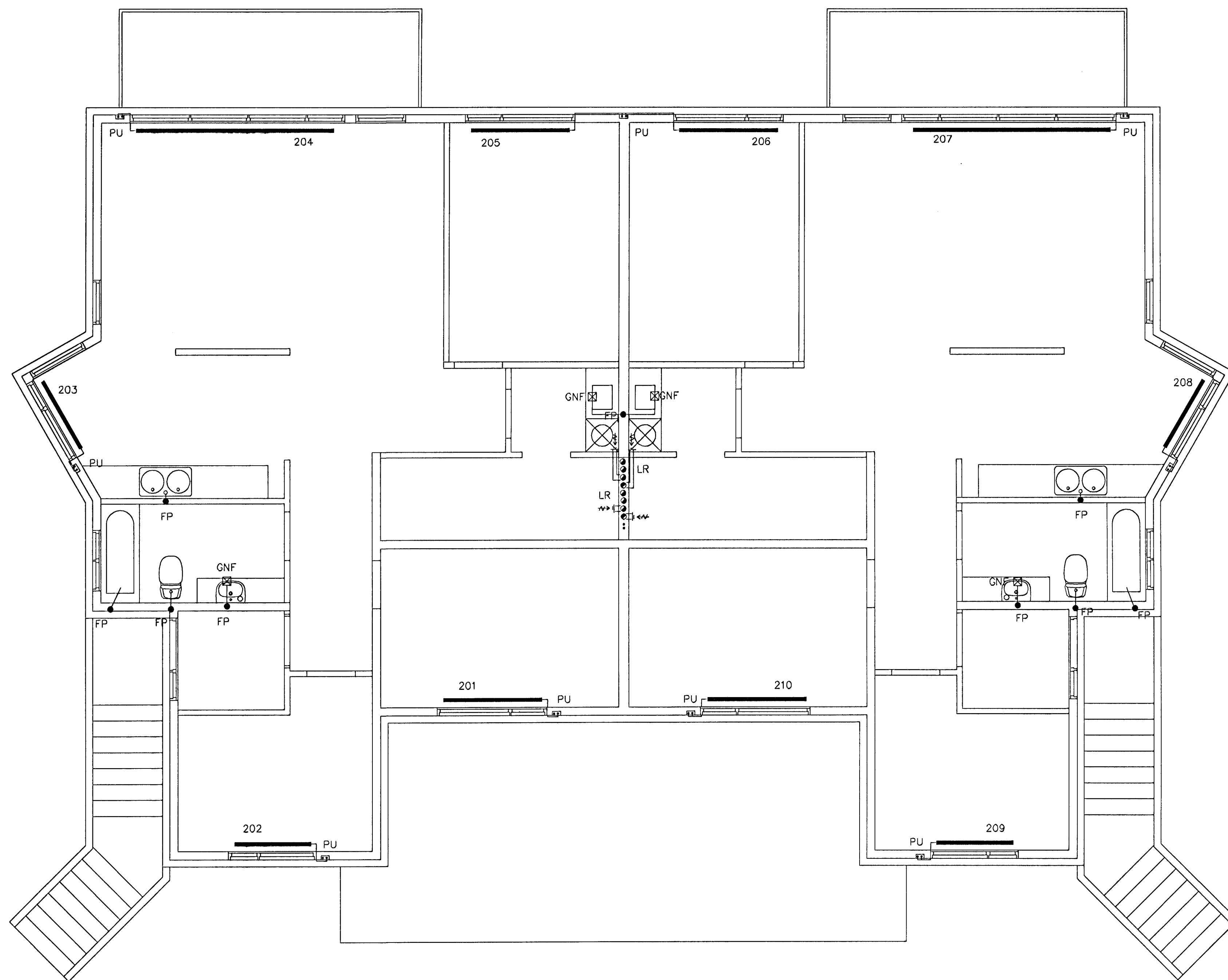
GRUNNMYND 2 HÆÐAR 1:50
