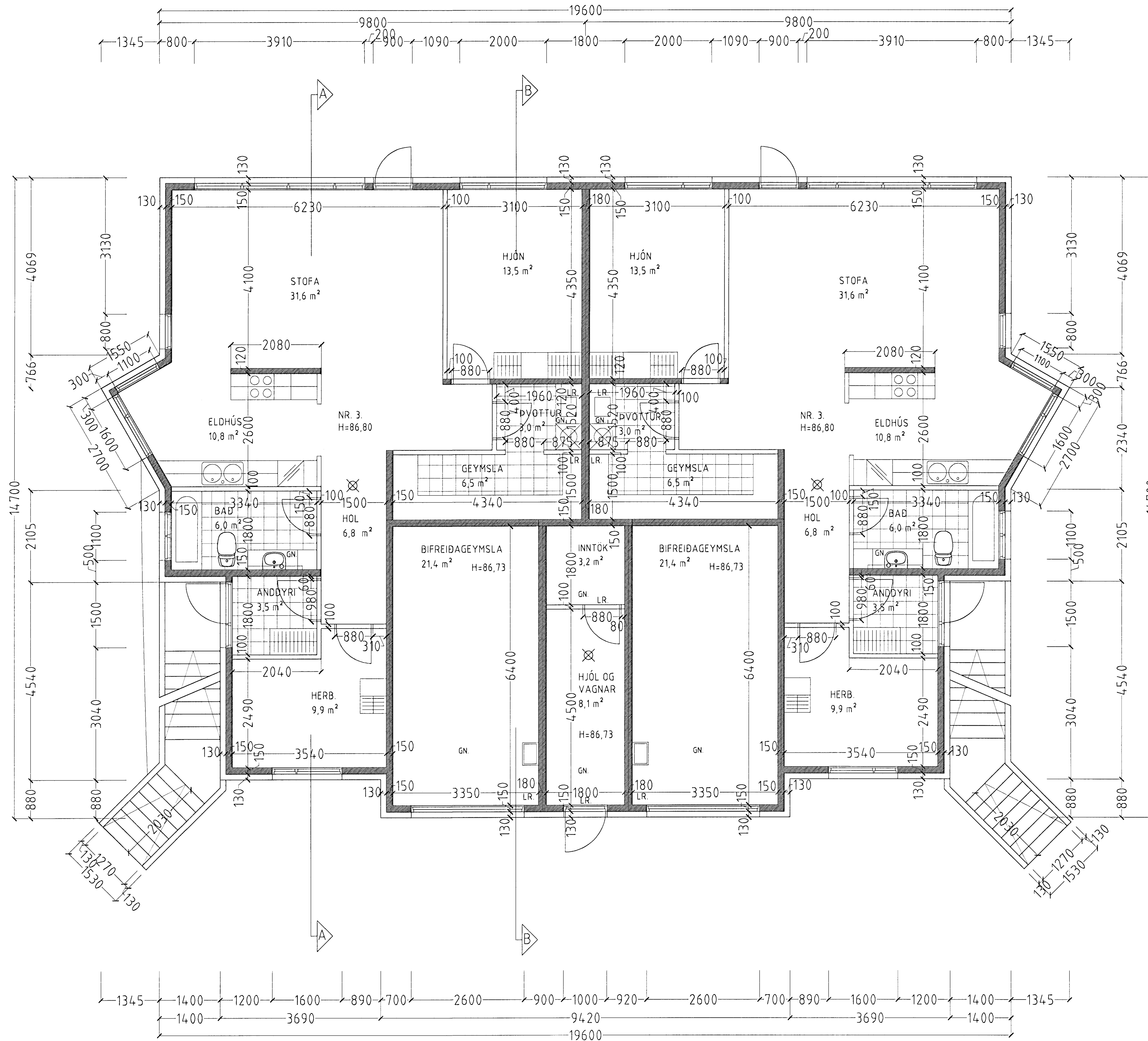
GRUNNMYND 1. HÆÐ MKV. 1:50.
