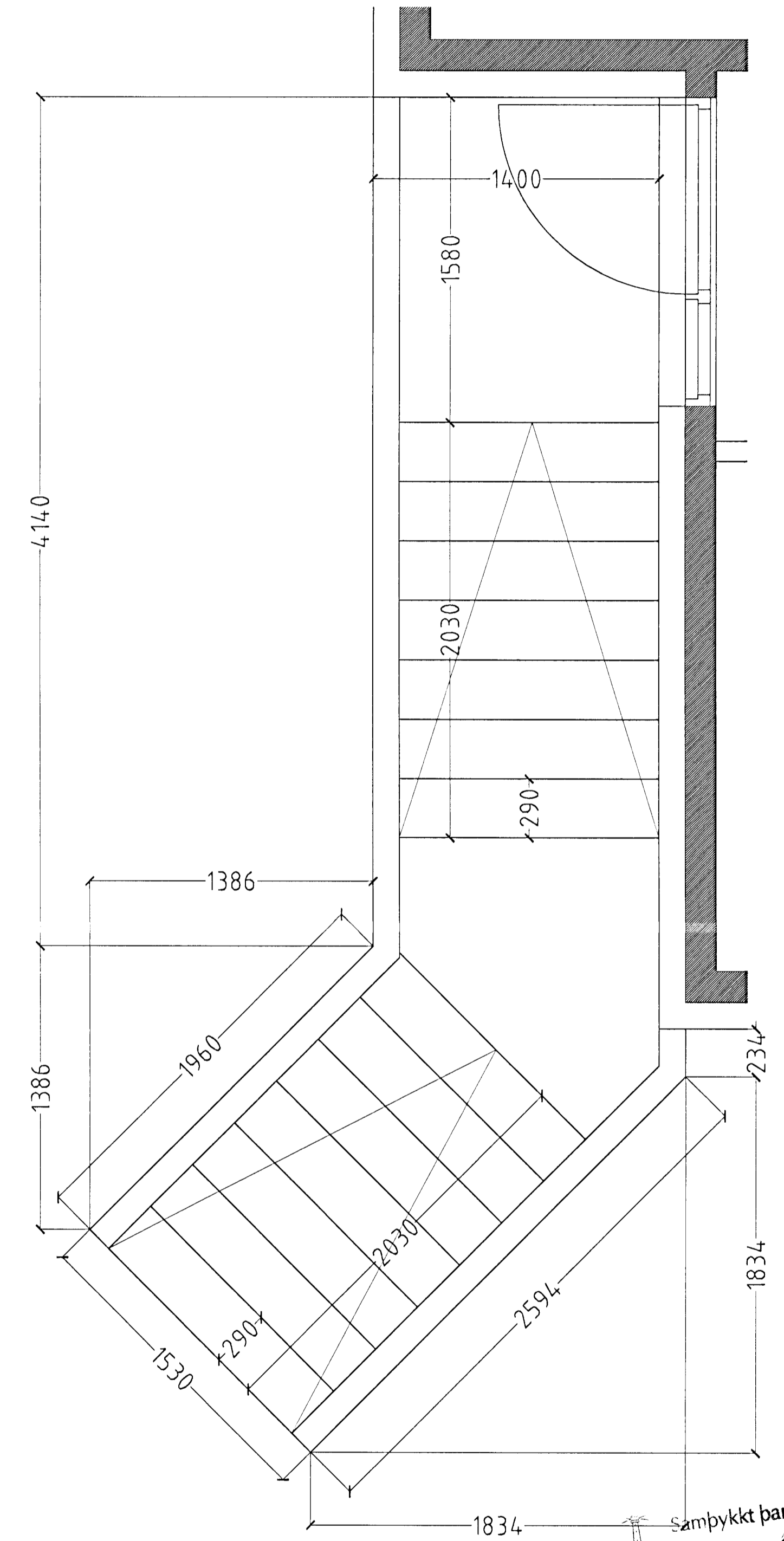
GRUNNMYND STIGI MKV. 1:20.
