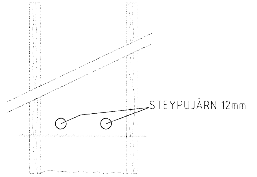
SNÍÐ AF STEYPUÞEINUM Í SÖKKLUM ENGINN MÆLIKVARÐI
