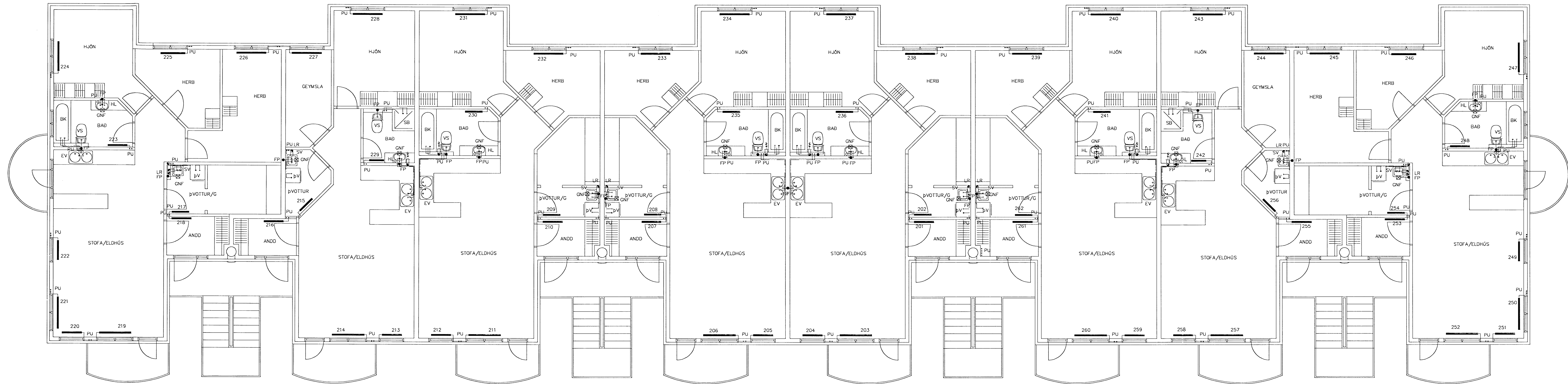
GRUNNMÝND 2 HÆÐAR 1:50
