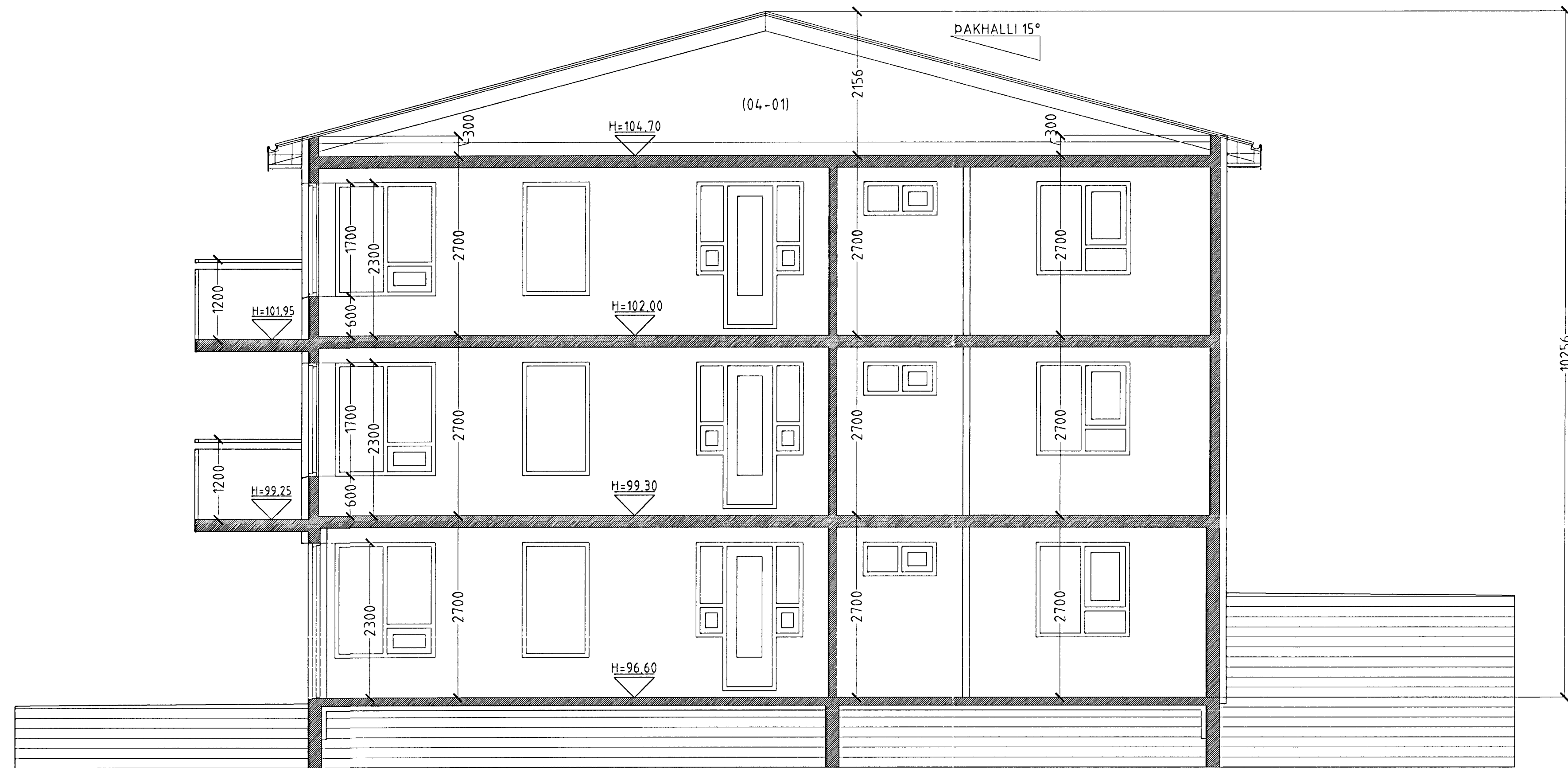
SNID A-A MKV. 1:50.
