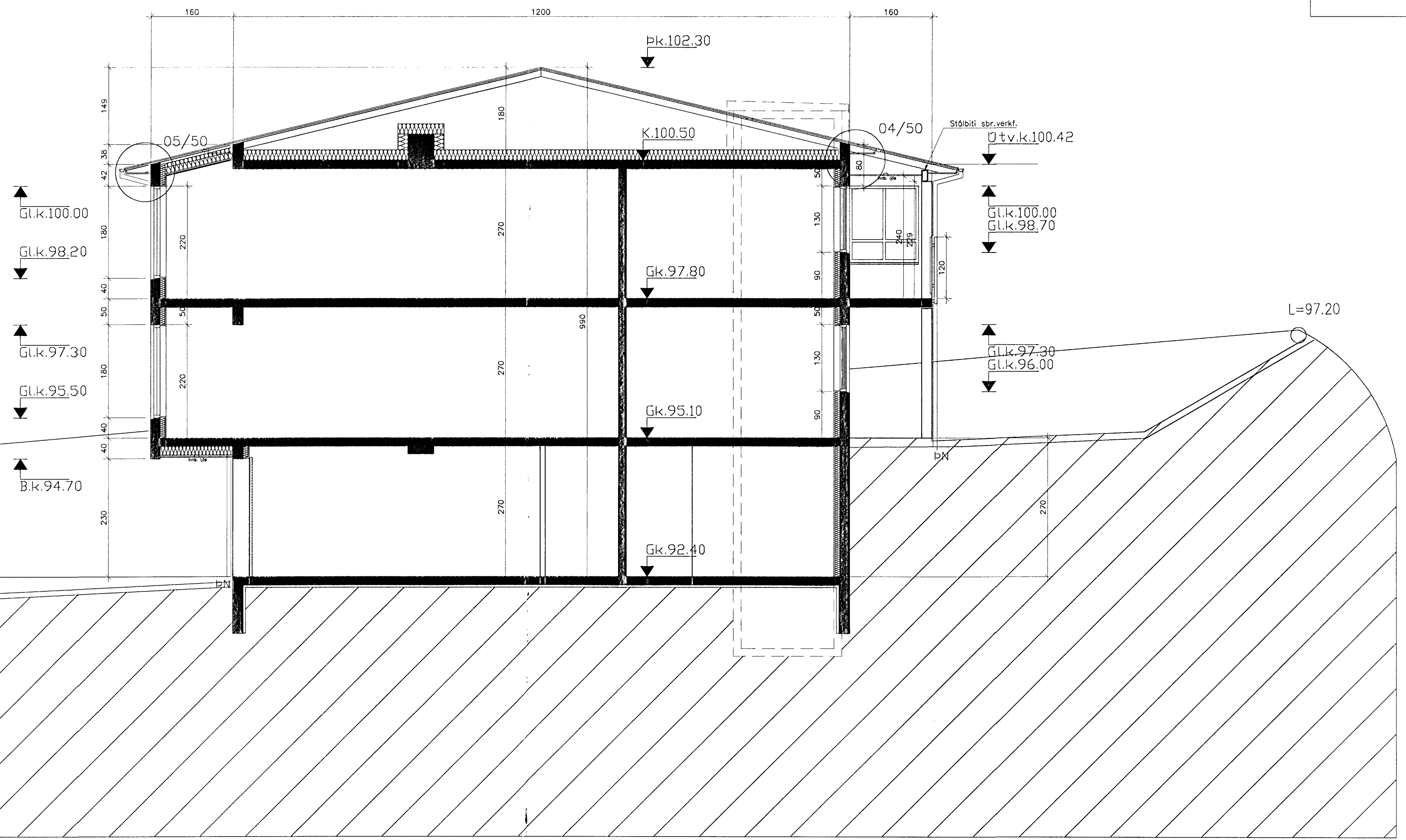
SNEIÐING A-A
