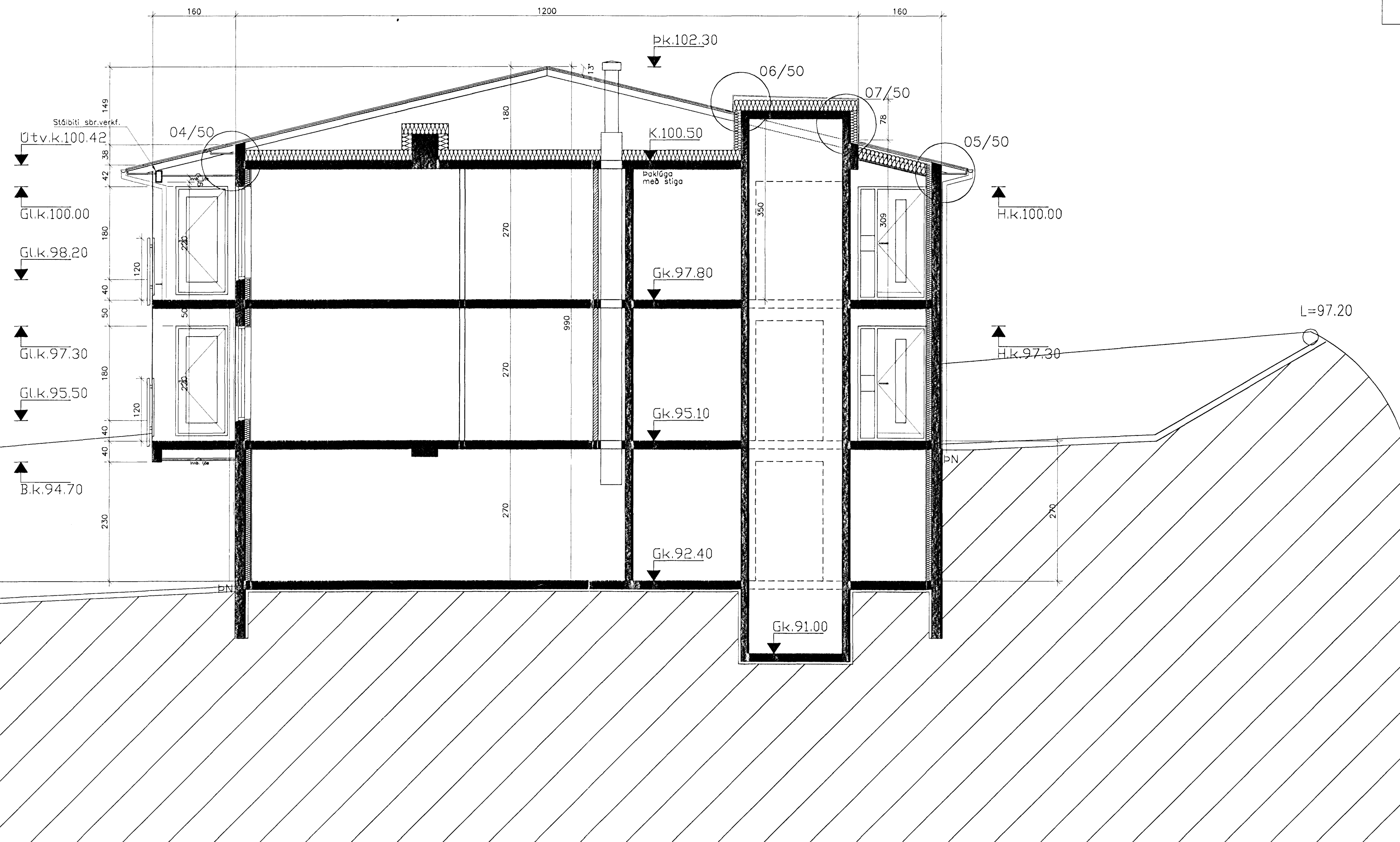
SNEIDING B-B
