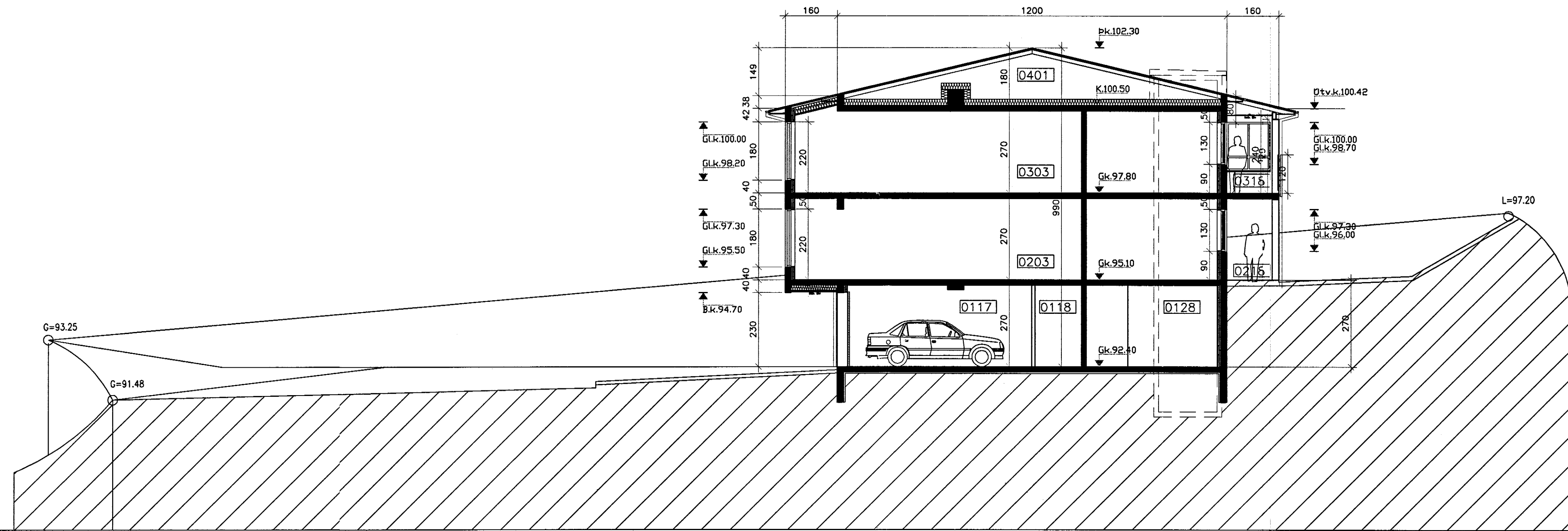
SNEIDING A-A
