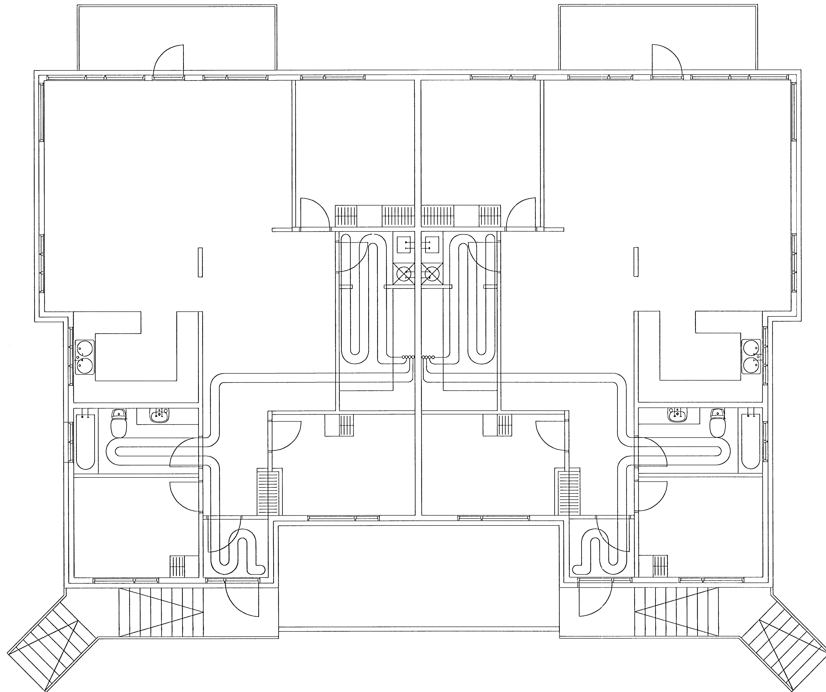
GRUNNMYND 2 HÆÐAR 1:50
