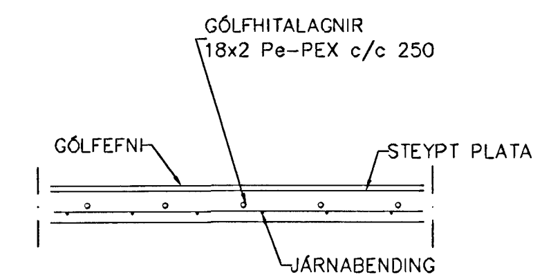
GÓLFHITI SNIB, 1:20
