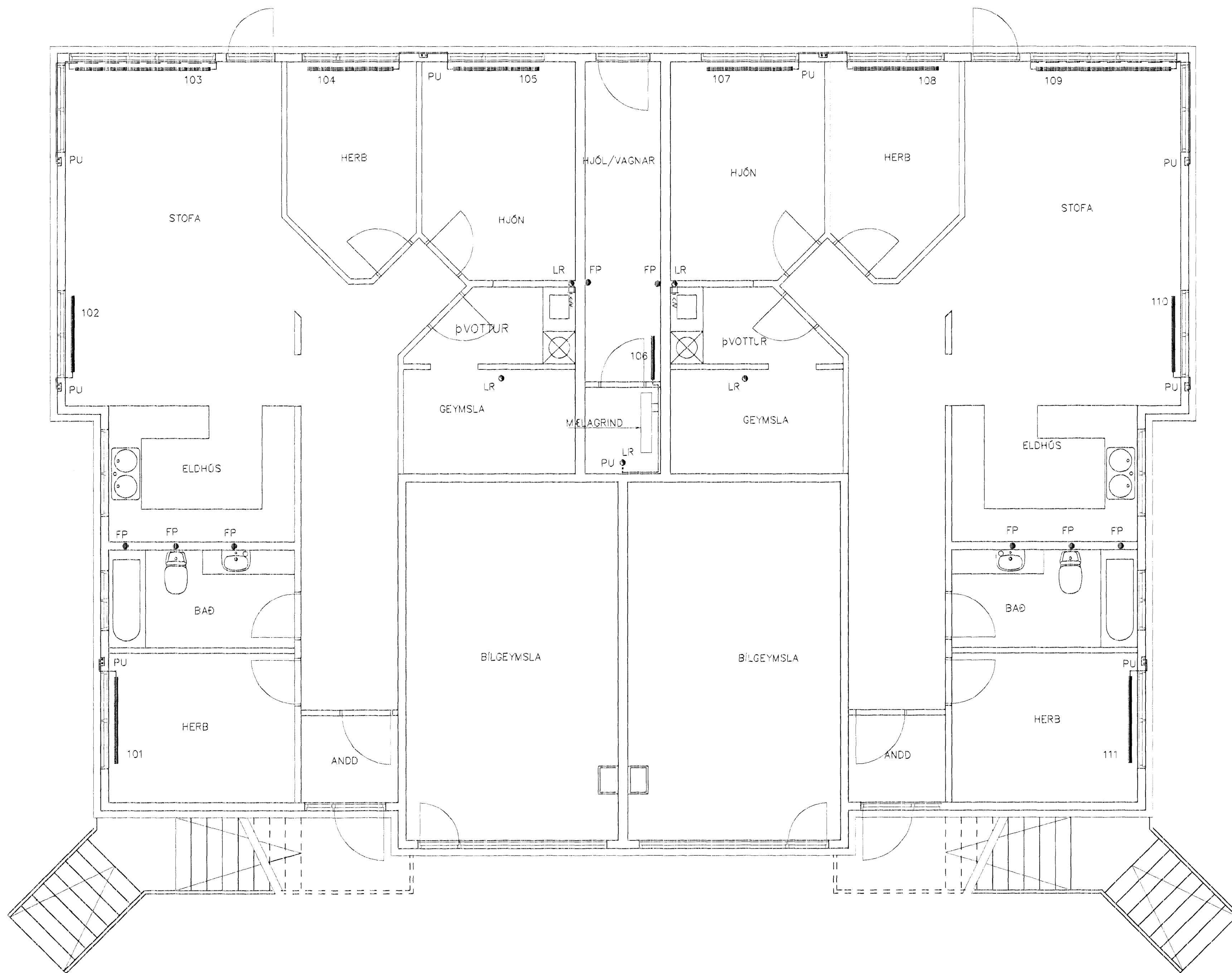
GRUNNMYND 1 HÆÐAR 1:50
