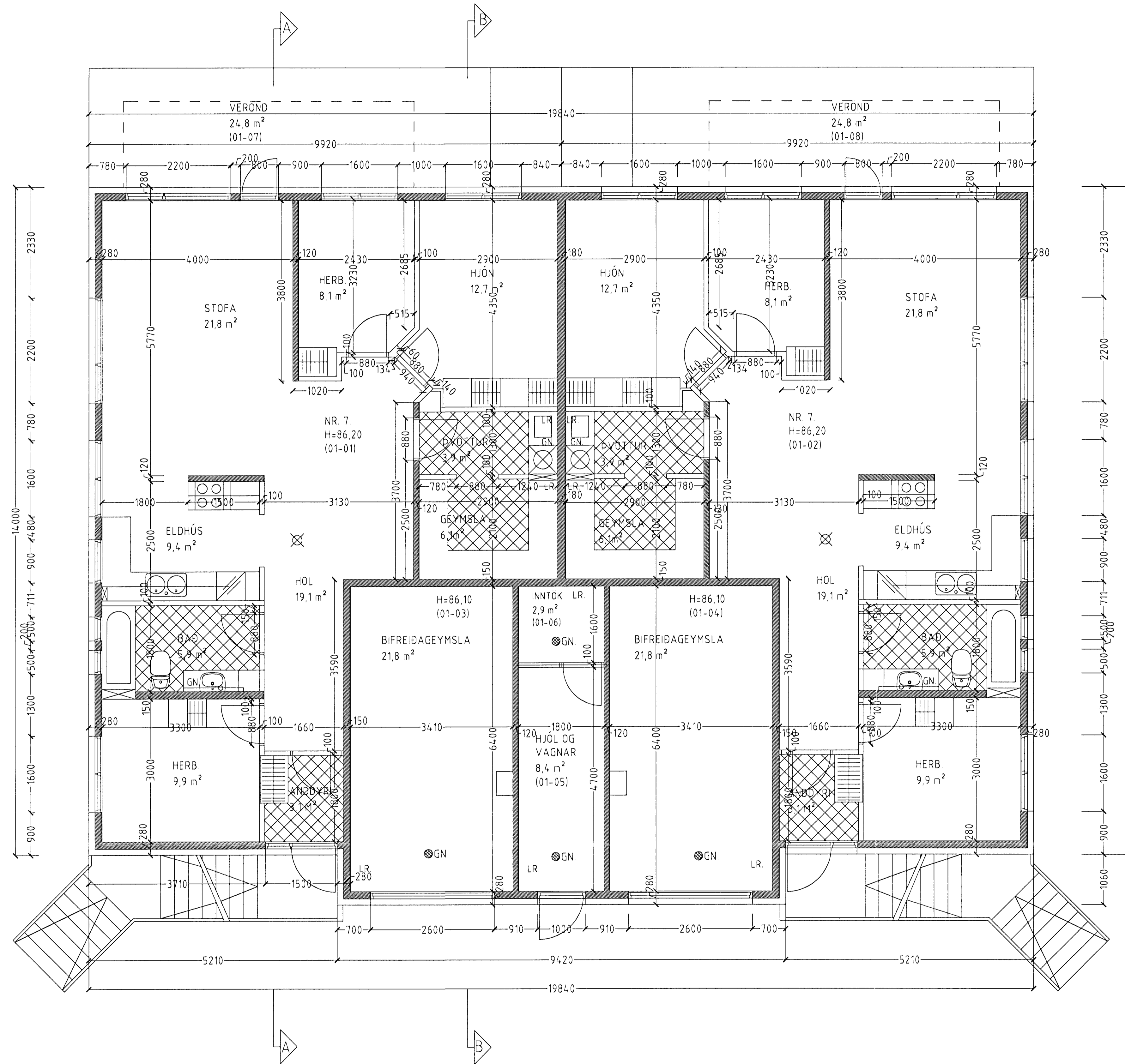
GRUNNMYND 1 HÆÐ MKV. 1:50.
