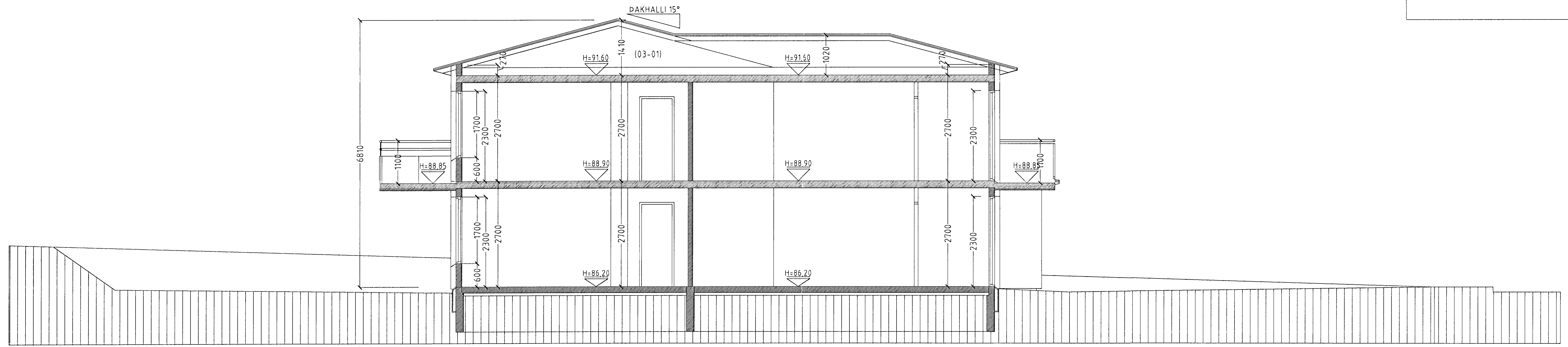
SNID A-A MKV. 1:50.
