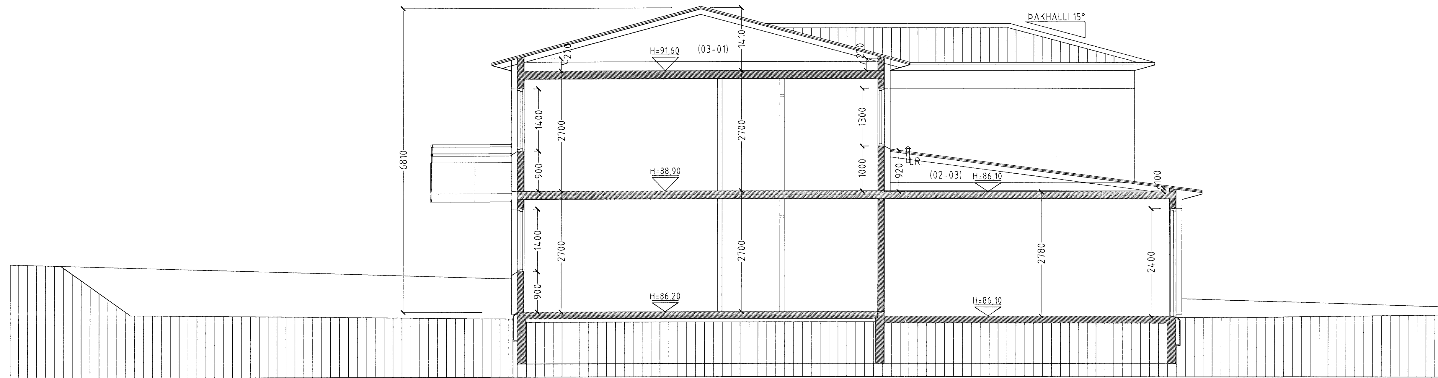
SNID B-B MKV. 1:50.
