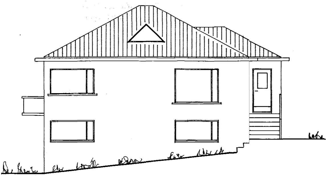
SUÐUR
