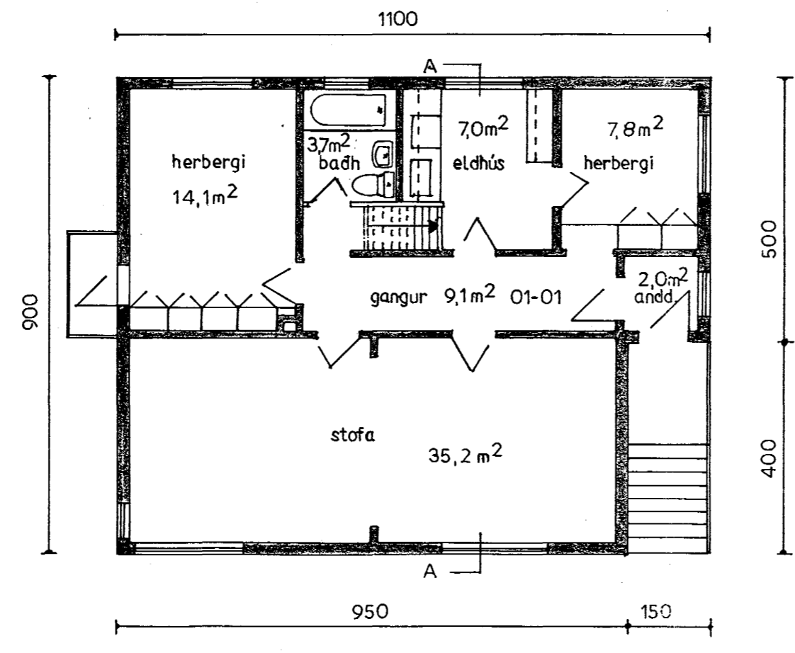
I HÆÐ
