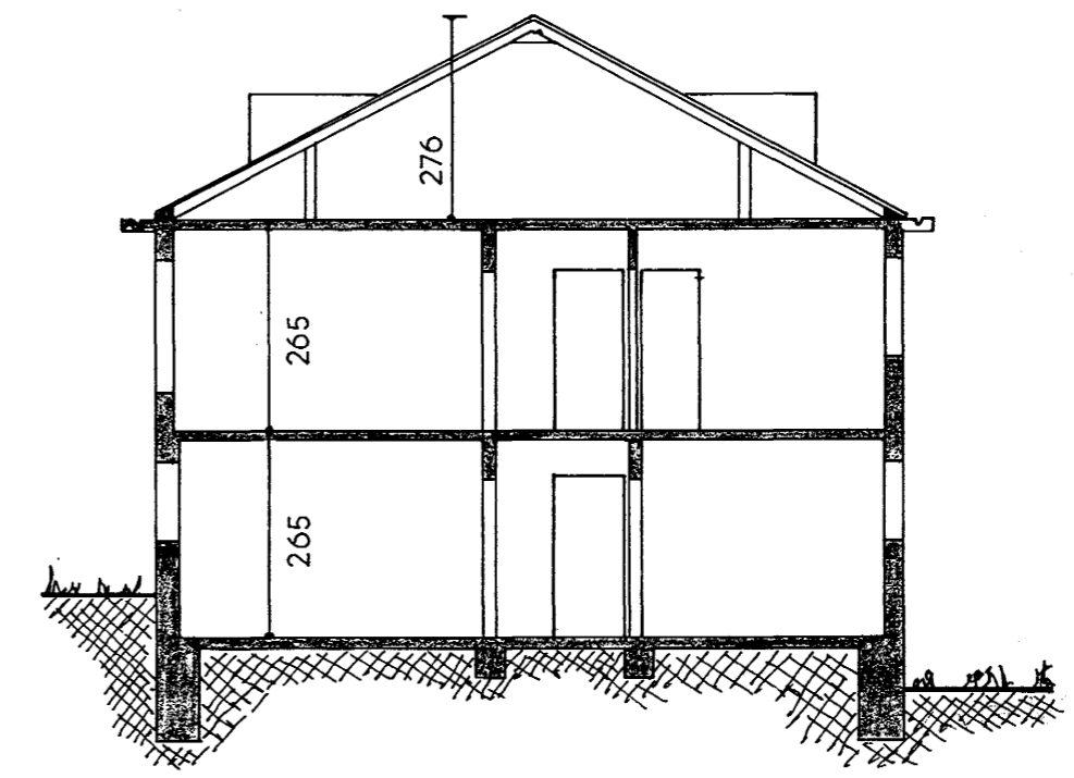
SNIÐ A-A
