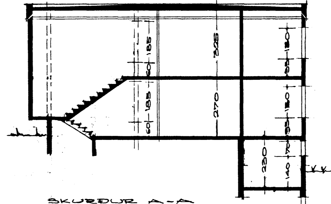
SKURÐUR A-A
