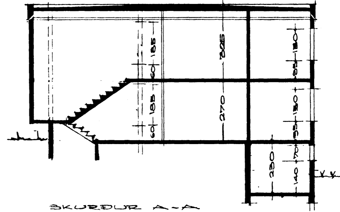
SKURÐUR A-A
