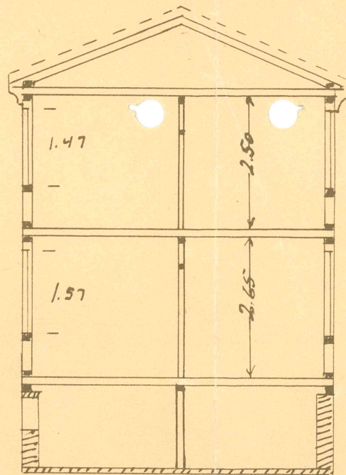
SKURÐUR N.B.
