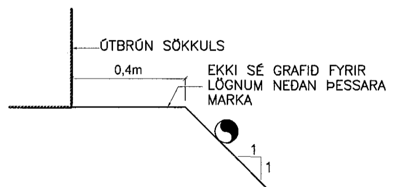
LEGA LAGNA VÍÐ HÚS 1:20
