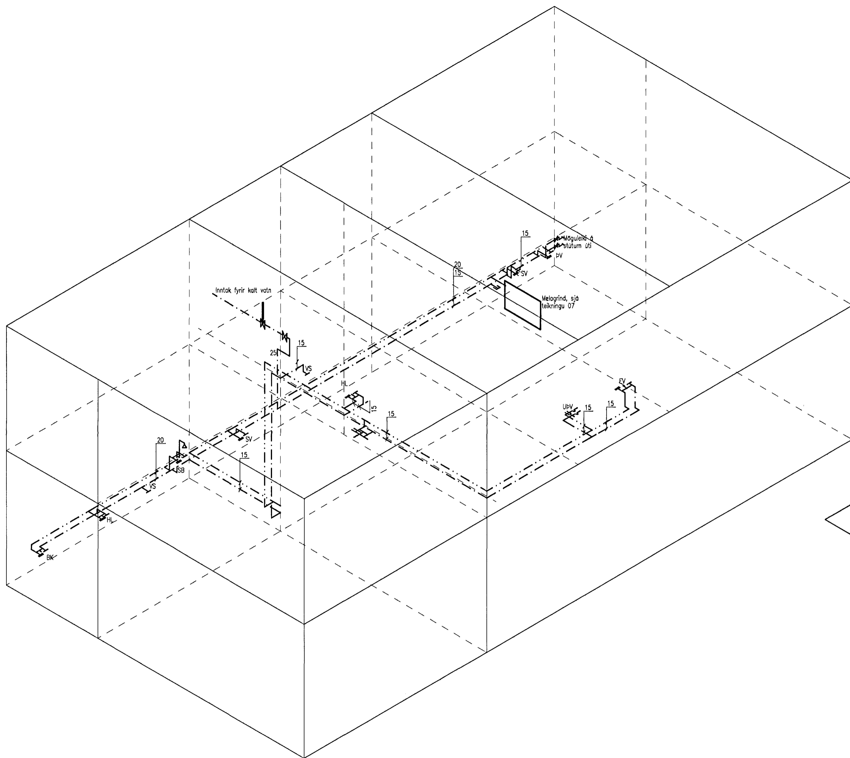
KERFISMYND VATNSLAGNA 1:50
