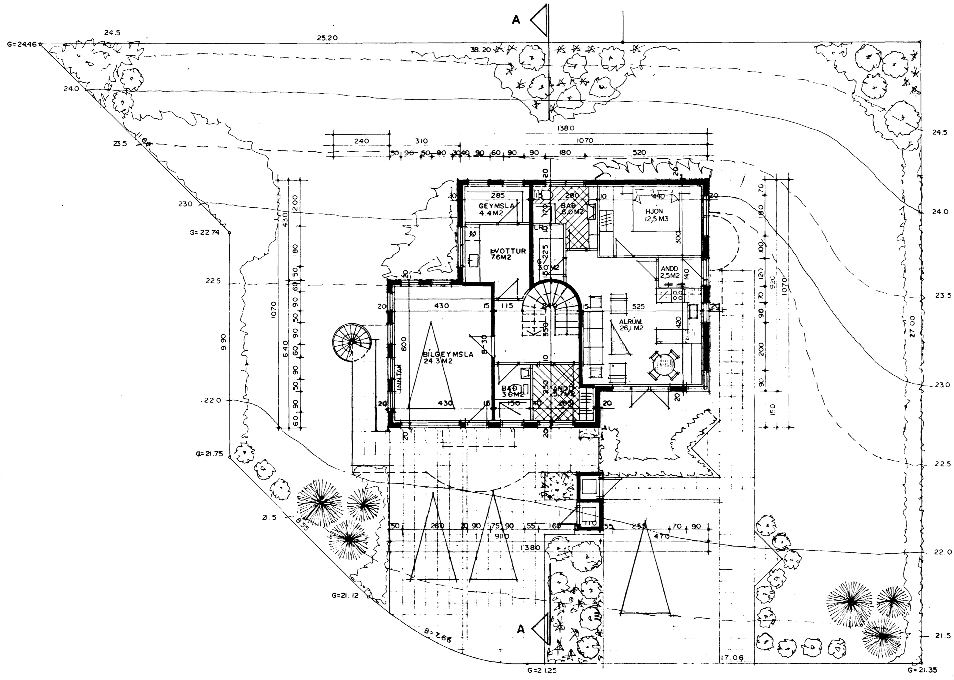
GRUNNMYND I. HÆÐAR MKV 1:100
