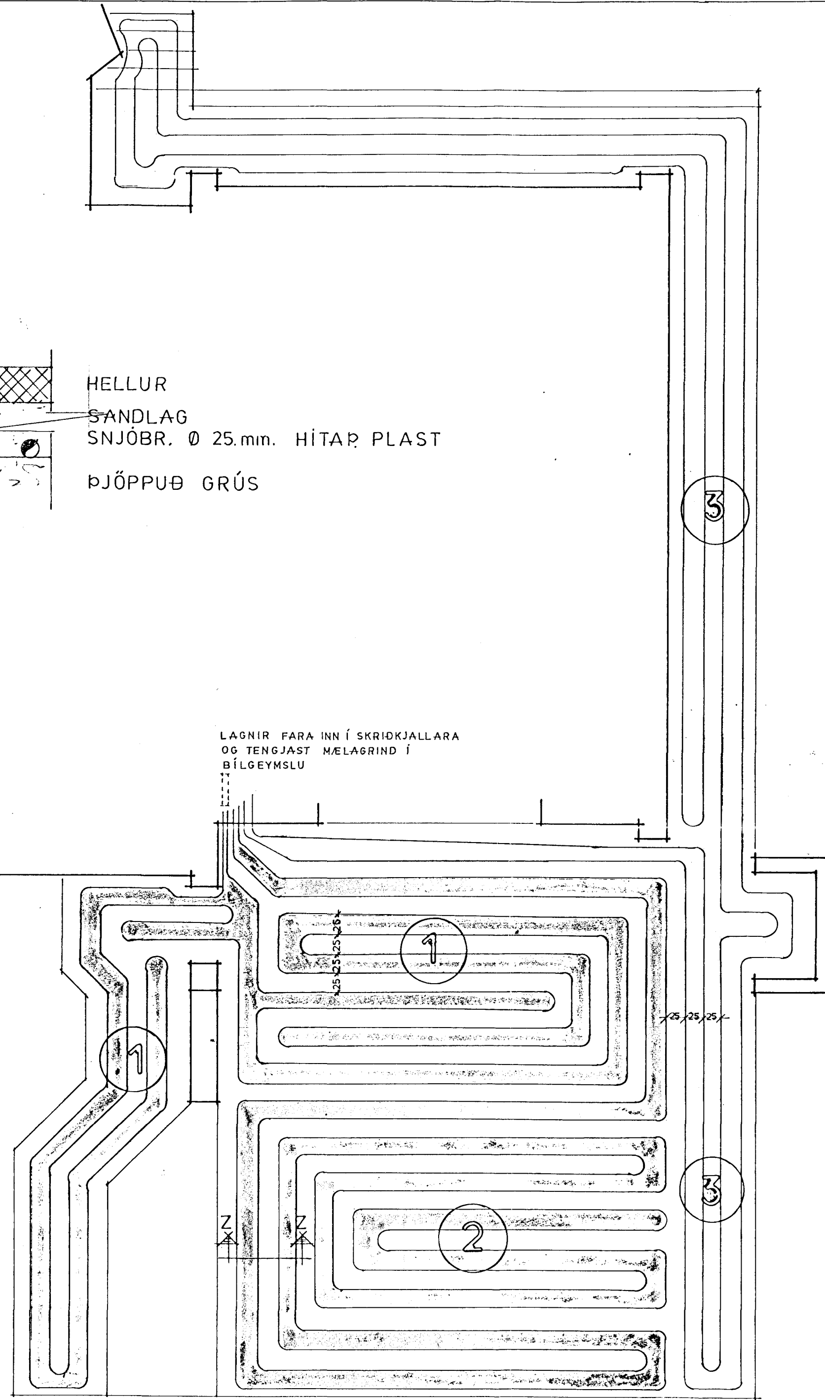
GRUNNMYND 1:50
